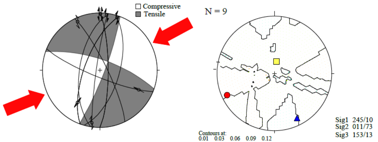
Slika 5-14. Stereografska projekcija orijentacije i vektora pomaka rasjeda i smičnih pukotina duž pružanja strike-slip rasjeda izmjerenih u području poligona Plitvički rasjed.
