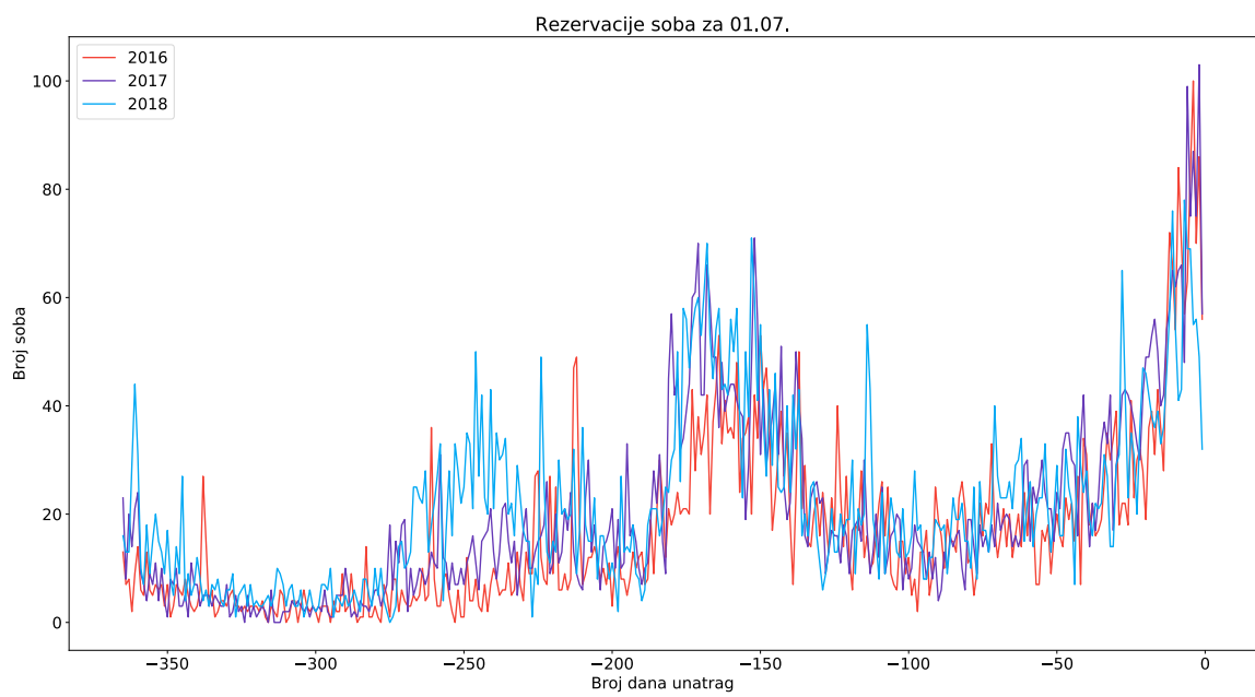
Slika 3.2: Sezonálnost vremenskog niza rezervacija
