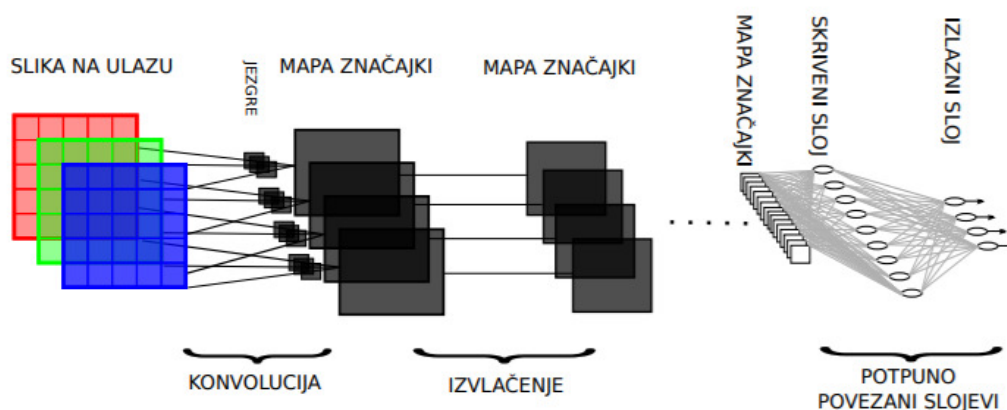
Slika 8.8: Convolutional neural networks - CNN (preuzeto iz [4])
