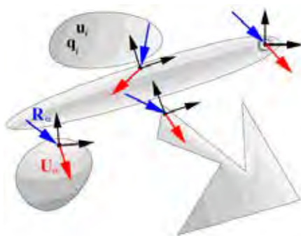
Slika 1. Četiri različita tijela za primjenu u SOLFEC računalnom kodu (Koziaara, 2010)
