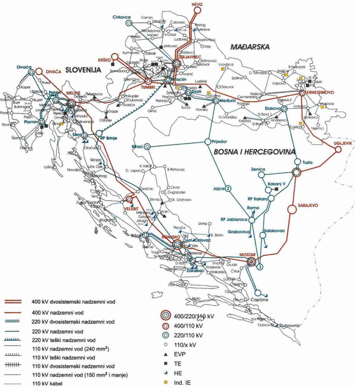
Slika 1. Prikaz modela prijenosne mreže Hrvatske s okruženjem korištenog u proračunu
