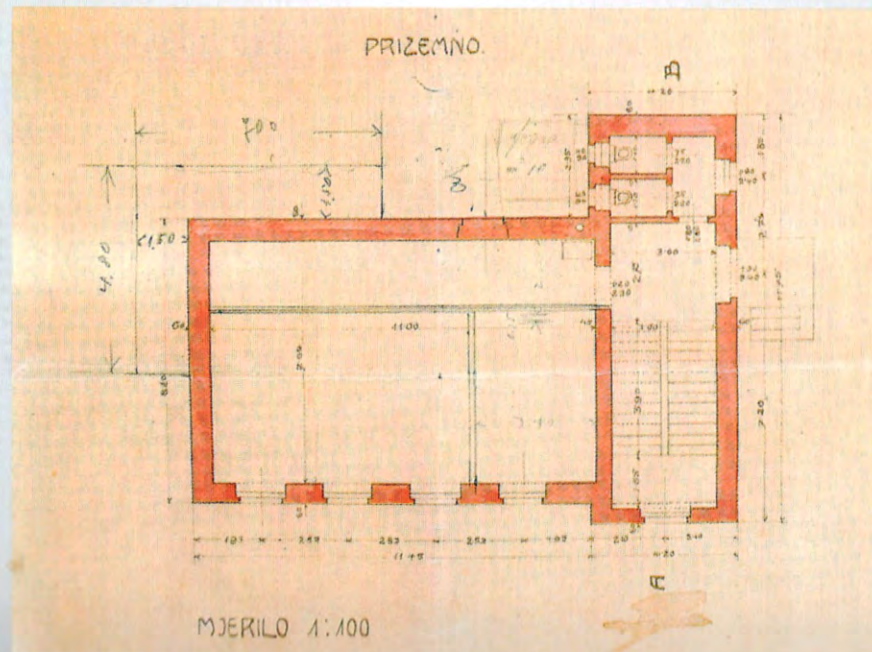
Nacrt prizemlja zgrade sa skiciranim preinakama za dodavanje otpadne jame
