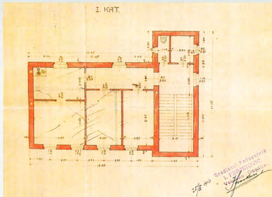
Tloris 1. kata s pečatom i potpisom I. Frankovića iz 1913. godine
