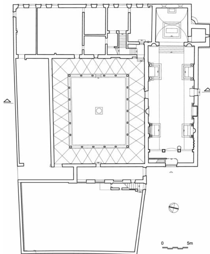
Poprečni presjek i tlocrt crkve sa samostanom
