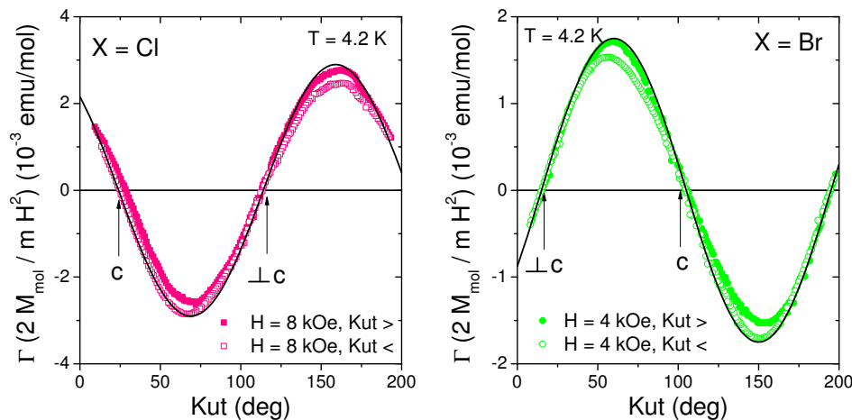
Slika 6.8 – Kutna ovisnost magnetskog momenta sile u uređenom stanju u \text{Cu}_2\text{Te}_2\text{O}_5\text{X}_2 ( \text{X}=\text{Cl} , \text{Br} ) u ravnini koja sadrži os c pri T = 4.2\text{K} . Crne linije predstavljaju pravilne sinusoide perioda 108^\circ . Kut > je oznaka za rotaciju polja od manjih k većim kutevima, a Kut < obrnuto.
