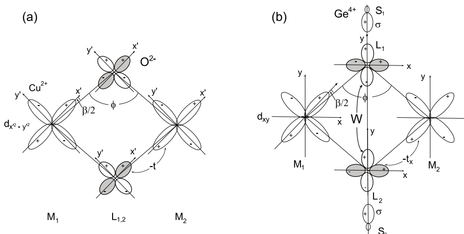
Slika 4.4 – Superizmjena u M-L-M klasteru ( Cu-O-Cu u CuGeO_3 ) sa i bez pozitivnih iona sa strane [Geertsma i Khomskii 96]. a) Klaster od dva magnetska iona M i dva liganda L . \beta je kut odstupanja od 90^\circ . M_1-L_1-M_2 kut je \phi = \pi/2 + \beta . Prikazane su d_{x^2-y^2} orbitale iona M i p_{x'} i p_{y'} orbitale liganda L . Element matrice transfera između ligandne orbitale p i magnetske d orbitale je t . b) Isti klaster, ali sa pozitivnim ionima S_1 i S_2 sa strane Ge^{4+} u CuGeO_3 koje daju \sigma orbitale. Koordinatni sustav xy je zarotiran za 45^\circ u odnosu na x'y' pa su magnetske orbitale d_{xy} . t_x je transfer integral između d_{xy} i p_x , a W je transfer integral između dviju p_y orbitala na ligandima L_1 i L_2 .
