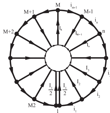
Slika 5.2.b Dodatne struje u kavezu pri prekidu štapa - parni broj štapova
