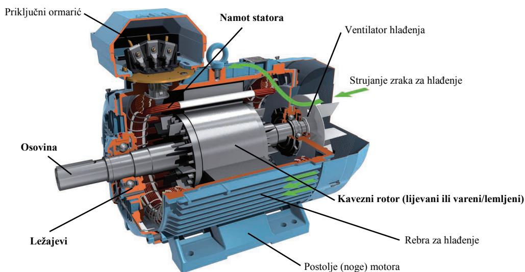
Slika 1.4. Konstrukcija suvremenog asinkronog kaveznog motora
