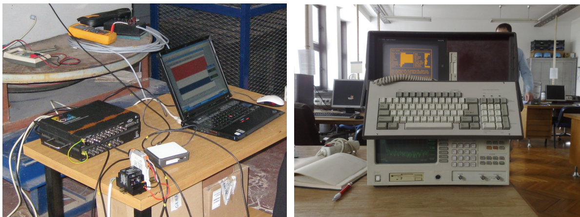
Slika F.1. Oprema za A/D pretvorbu i pohranu signala statorsche struje te spektralni analizator Hewlett Packard Dynamic Signal Analyzer 35665A CSA LR50254C
