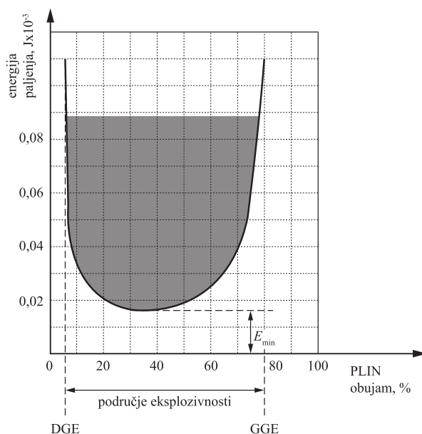
Slika 3.5. Granice eksplozivnosti smjese vodika ( \text{H}_2 ) i zraka
