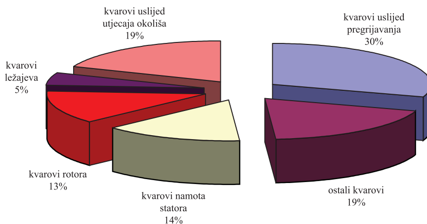
Slika 3.21. Učestalost kvarova asinkronog elektromotora [78]
