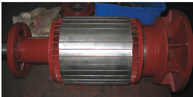
Slika 4.3. Kavez rotora elektromotora (380 V, 47 kW, Ex e II T1/T2/T3)
