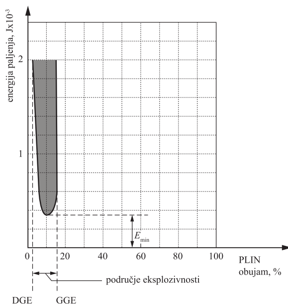
Slika 3.4. Granice eksplozivnosti smjese metana ( \text{CH}_4 ) i zraka
