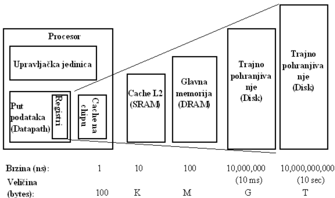
Sl. 2. Hijerarhijska organizacija memorijskog sustava današnjih računala (2) Izvor: FESB, Sveučilište u Splitu, Uvod u računalstvo- Računala i programiranje , http://laris.fesb.hr/index.html , (27.06.2004.)
