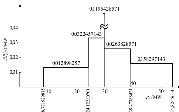
Figure 6 Probability density function of inflow- and outage-determined pumping capacity Slika 6. Funkcija gustoće vjerojatnosti dotokom i prekidom određenog pumpnog kapaciteta
