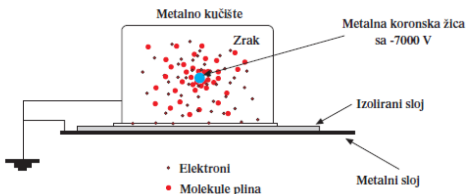
Slika 3 Schematski prikaz skorotrona
