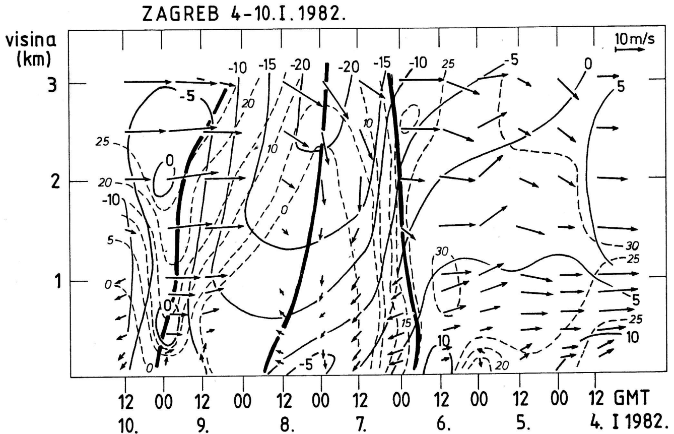
Sl. 7. Vremenski vertikalni presjek do 3 km visine nad Zagrebom za 4-10. 1. 1982. Vektori vjetra (u m/s) označeni su strelicom, tanje pune linije su izoterme (svakih 5°C), tanje isprekidane linije su izentropne \theta_e (svakih 5°C). Frontalne zone su označene debljim punim linijama.
