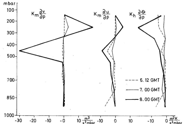
Sl. 10. Turbulentni tokovi momenta i topline nad Zagrebom za 6–8. 1. 1982.
