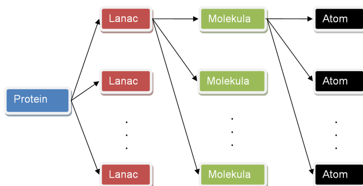
Slika 2.1: Struktura biomolekule
