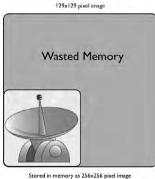
Slika 1. Neiskorištena memorija
