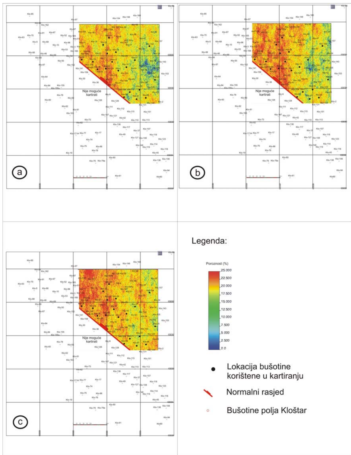
Slika 9.4: Distribucija poroznosti ležišta T kartirana sekvencijskim Gaussovima simulacijama: a -prva realizacija, b -pedeseta realizacija i c -stota realizacija
