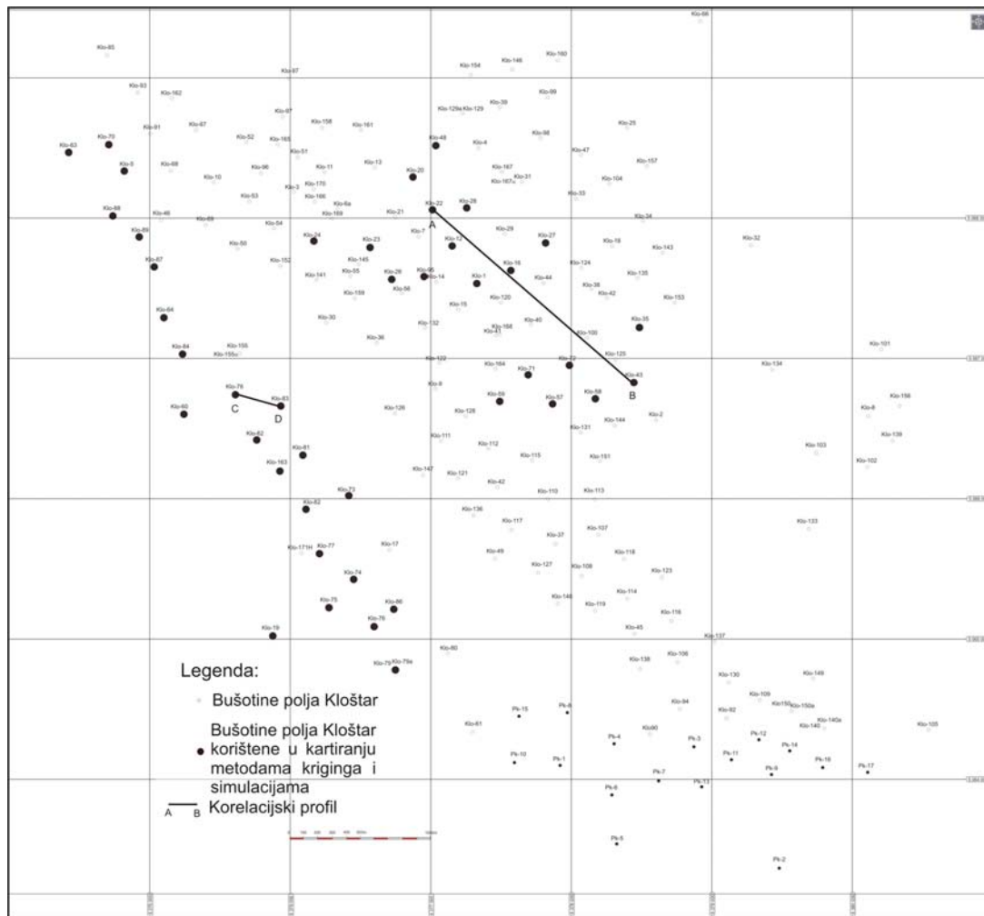
Slika 2.2: Karta lokacija bušotina na polju Klostar (VELIĆ et al., 2008*)
