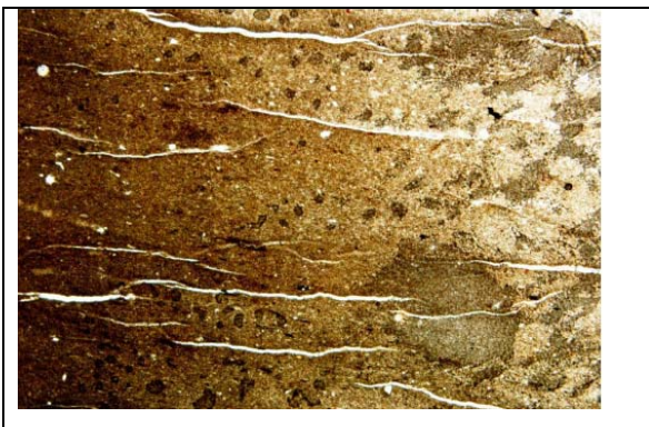
Slika 3.30: Lapor s otvorenom mikrofrakturnom poroznošću, (Klo – 12, 1071,0 – 1073,0 m, I. m) (autor TADEJ, J., iz studije: VELIĆ et al., 2008*)
