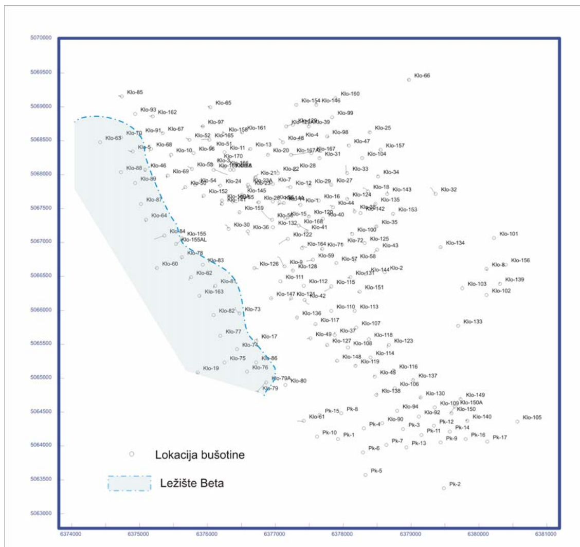
Slika 3.6: Današnji položaj gornjopanonskog ležišta Beta
