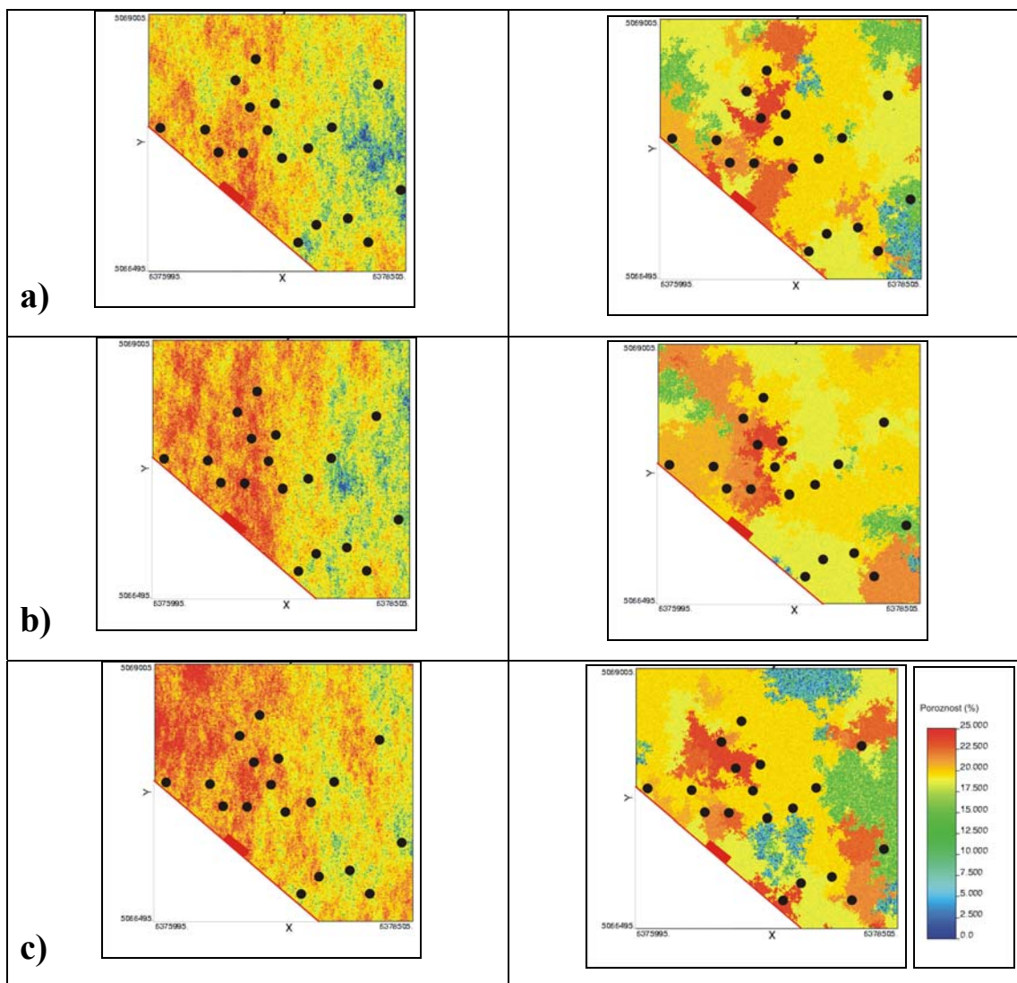
Slika 9.30: Usporedba realizacija distribucije poroznosti ležišta T dobivenih sekvencijskim Gaussovim simulacijama (lijevo) i sekvencijskim indikatorskim simulacijama (desno): a) prva realizacija, b) pedeseta realizacija i c) stota realizacija
