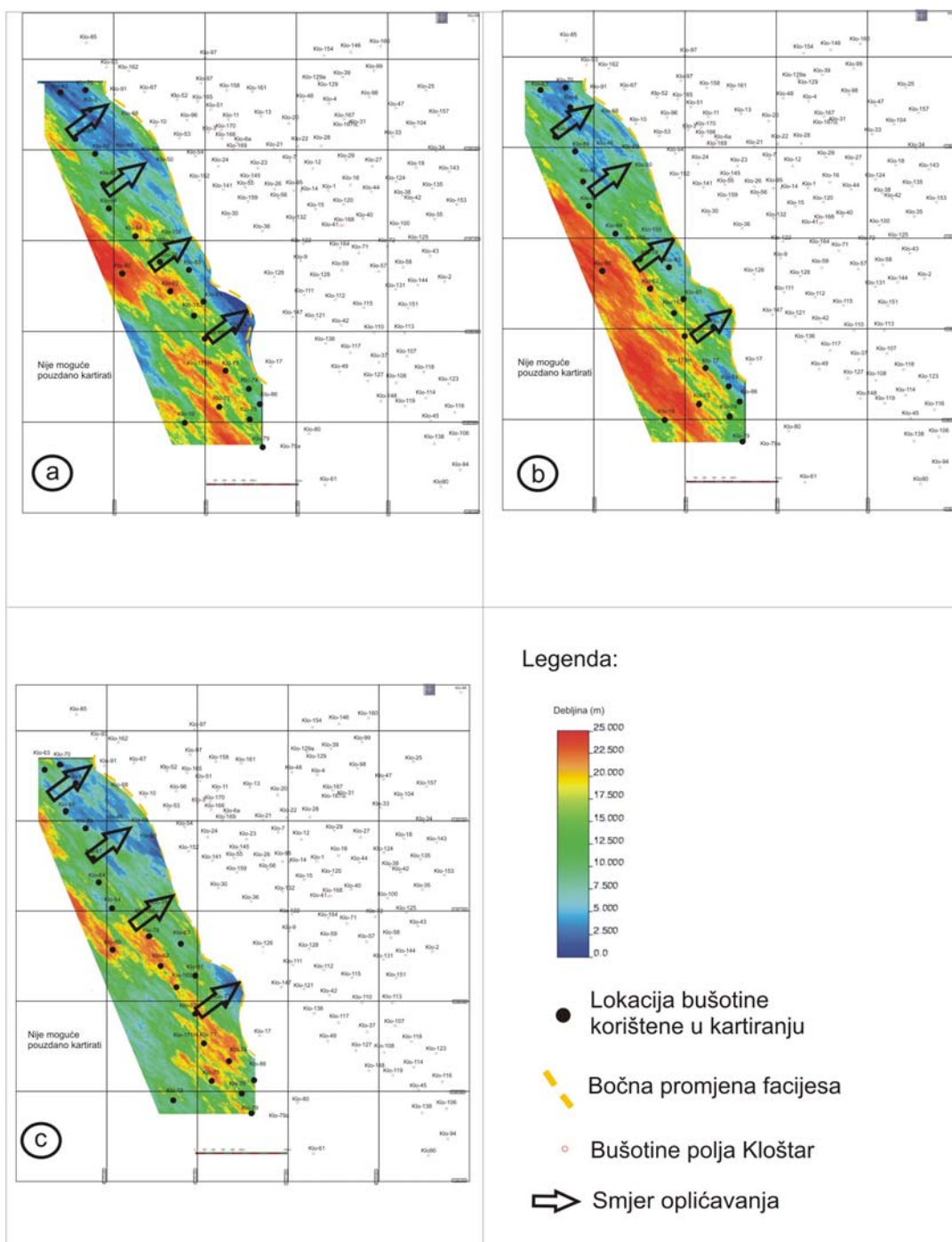
Slika 9.2: Distribucija debljine ležišta Beta kartirana sekvencijskim Gaussovim simulacijama: a-prva realizacija, b-pedeseta realizacija i c-stota realizacija
