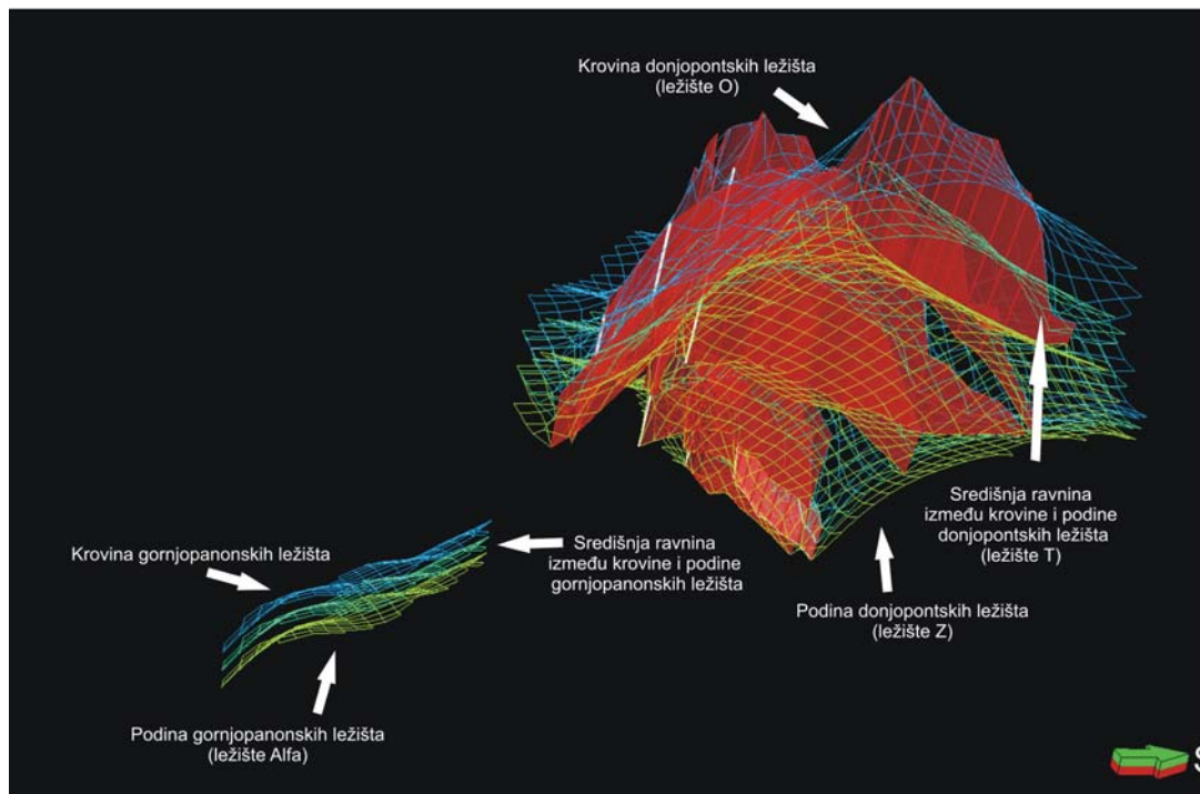
Slika 7.11: Temeljni strukturalni model gornjopanonskih i donjopontskih ležišta
