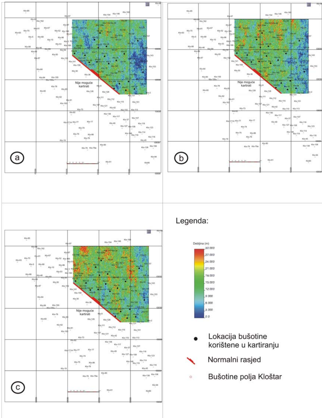
Slika 9.5: Distribucija debljine ležišta T kartirana sekvencijskim Gaussovima simulacijama: a -prva realizacija, b -pedeseta realizacija i c -stota realizacija
