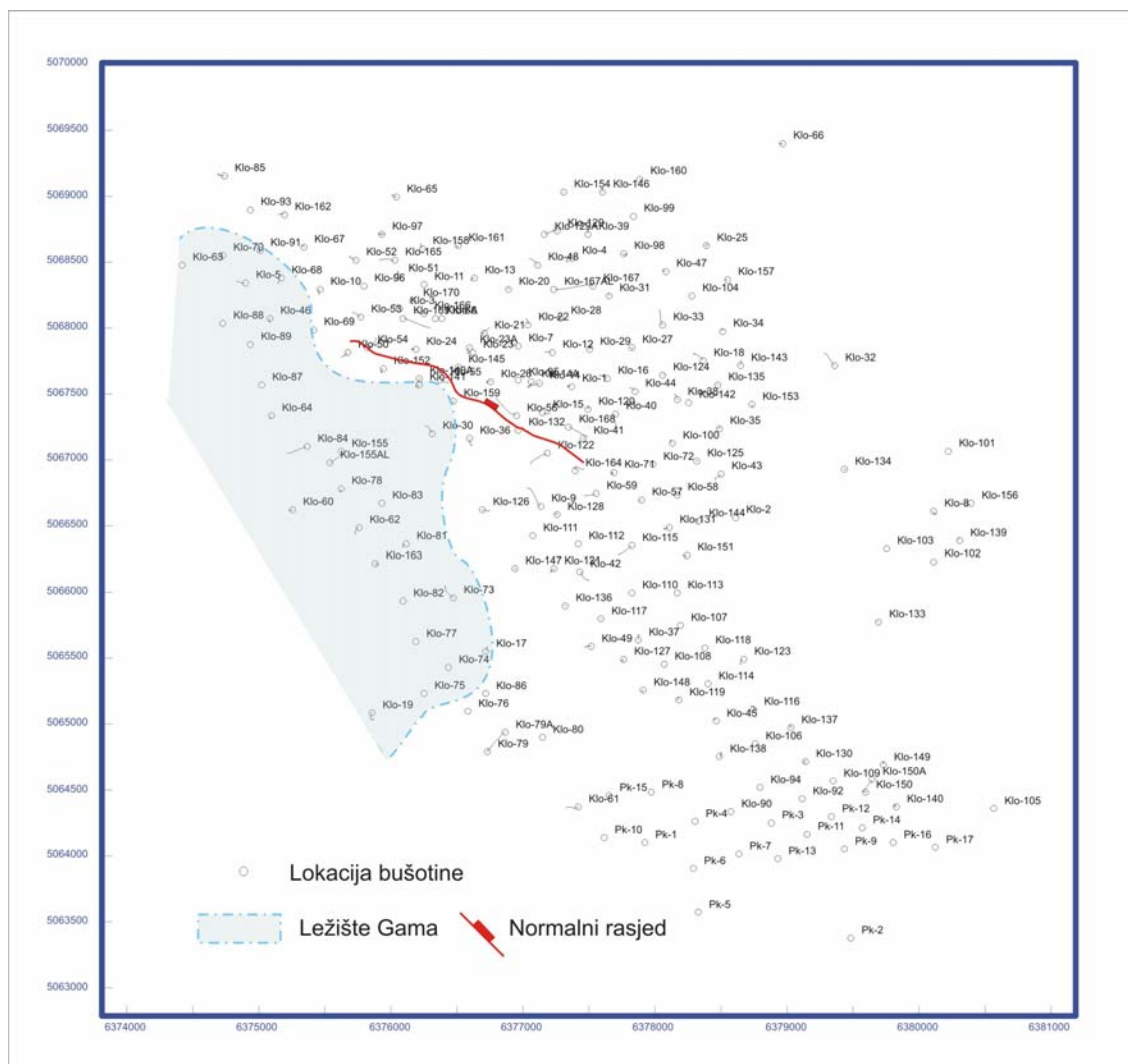
Slika 3.7: Današnji položaj gornjopanonskog ležišta Gama
