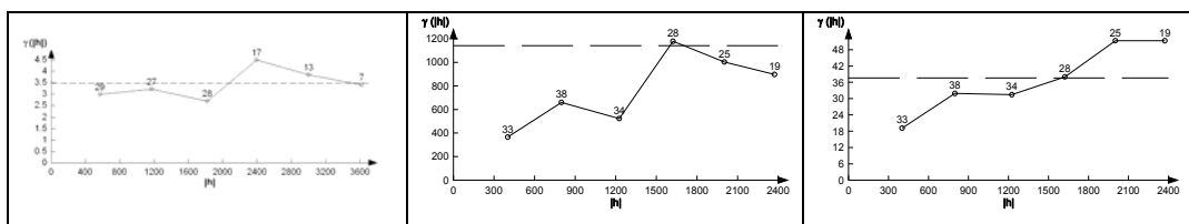
Slika 8.3: Eksperimentalni variogrami poroznosti (lijevo), dubine (sredina) i debljine (desno) gornjopanonskog ležišta Beta
