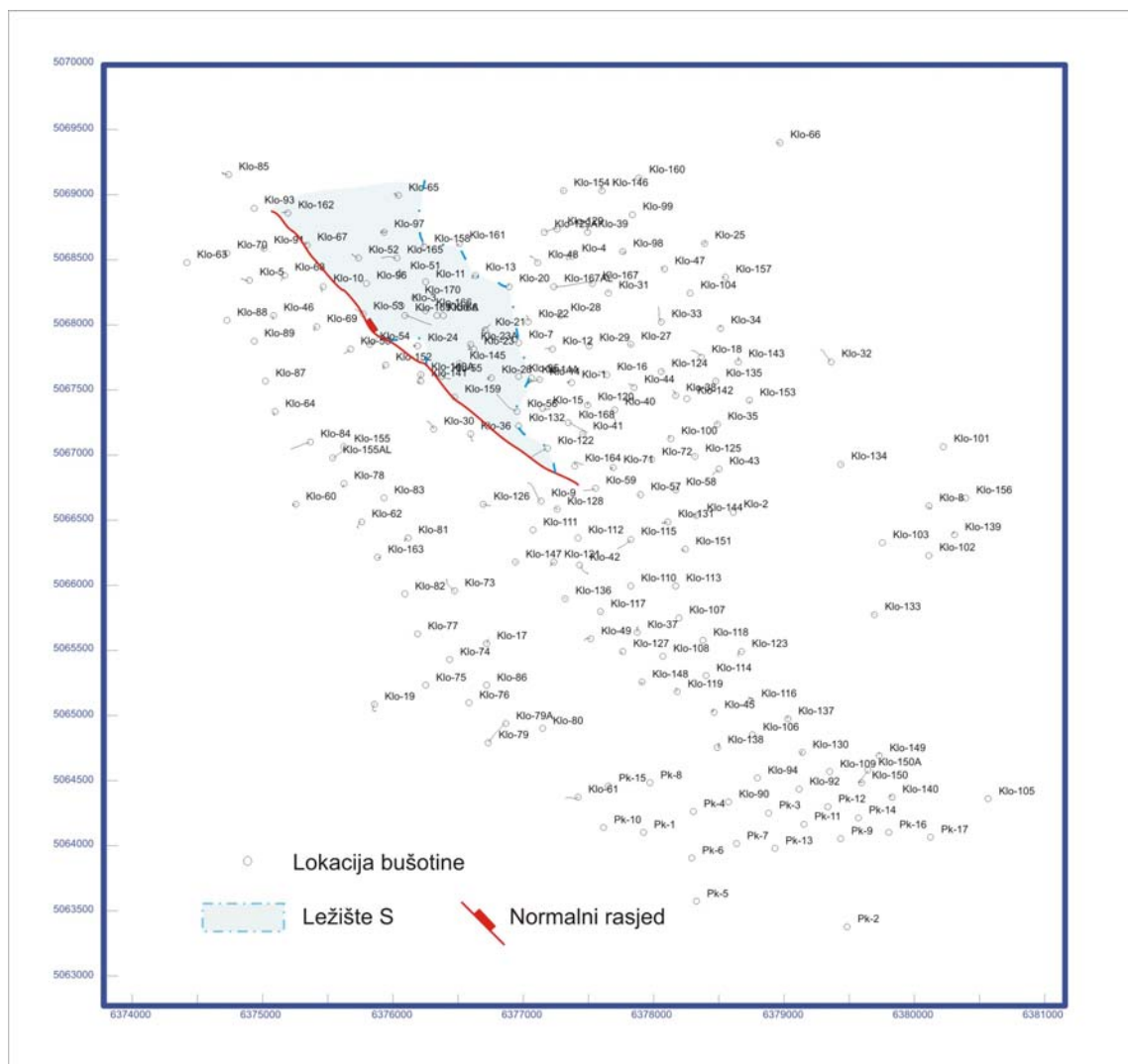
Slika 3.18: Današnji položaj donjopontskog ležišta S
