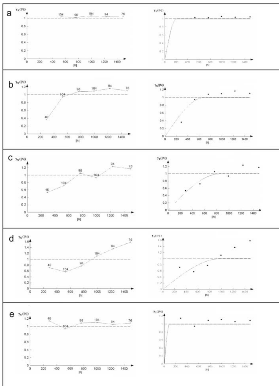
Slika 8.23: Eksperimentalni variogrami (lijevo) te njihova aproksimacija teorijskim krivuljama (desno) varijable poroznosti ležišta T za granične vrijednosti: a-14%, b-18%, c-19%, d-20% i e-22%.
