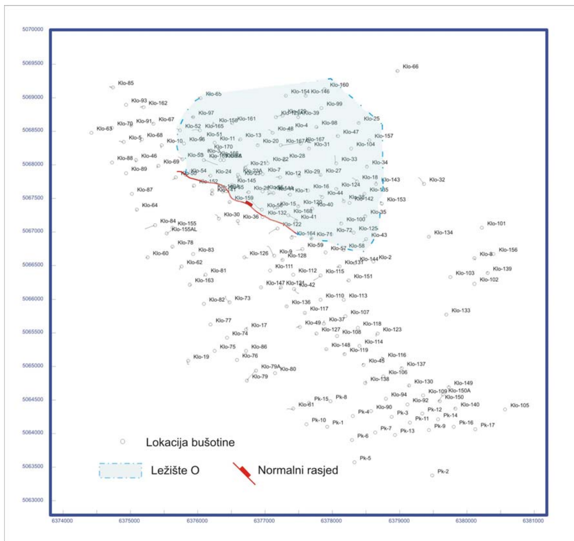
Slika 3.22: Današnji položaj donjopontskog ležišta O
