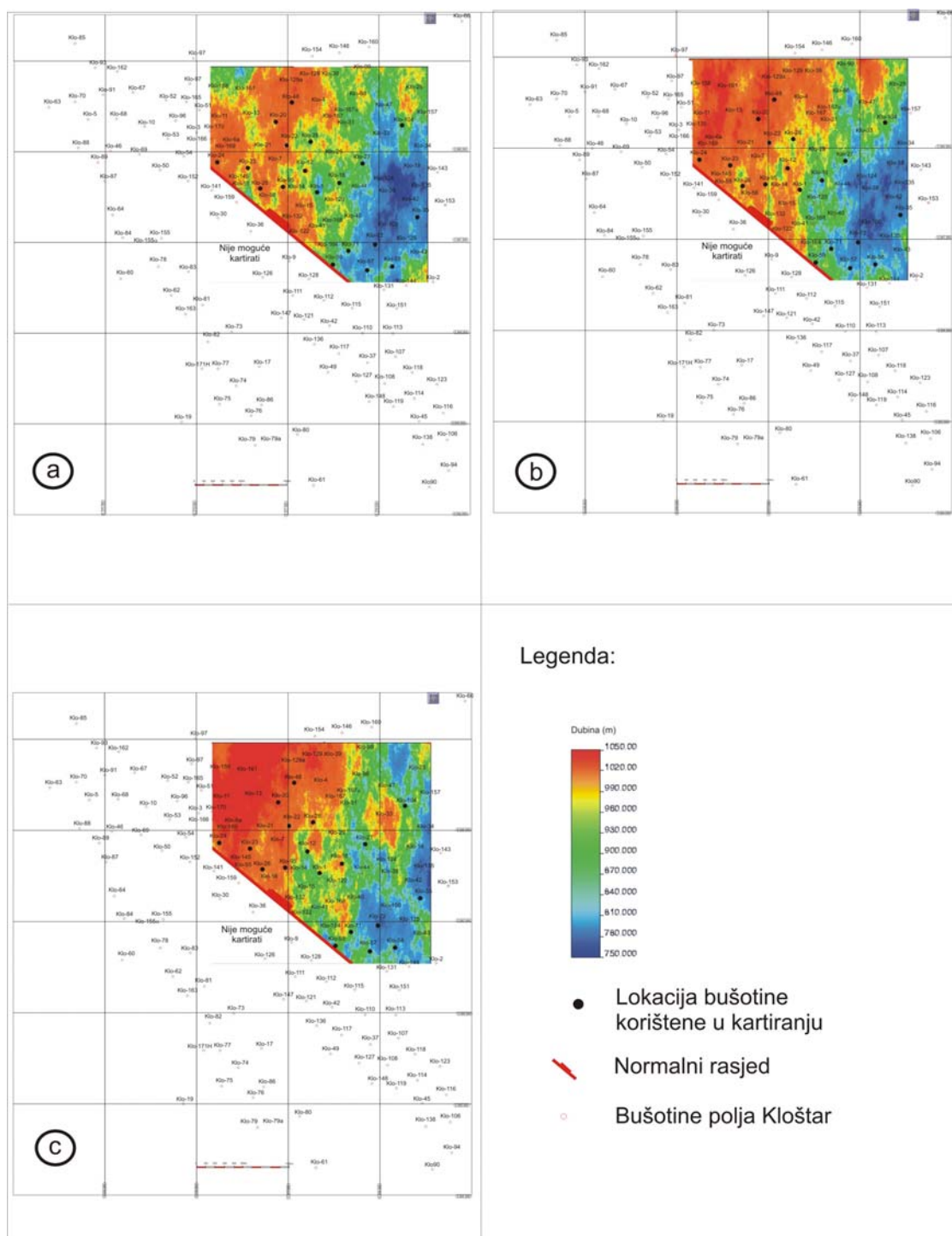
Slika 9.6: Distribucija dubine ležišta T kartirana sekvencijskim Gaussovim simulacijama: a- prva realizacija, b-pedeseta realizacija i c-stota realizacija
