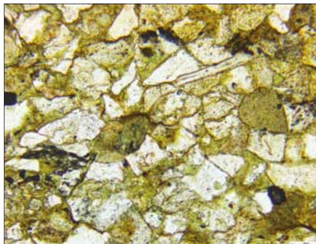
Sl. 200 Mikrofotografija litične grauivake (N=). Uzorak: SJ 1776-N 706 (veličina skale 100 mikrona), kat. br. 2
