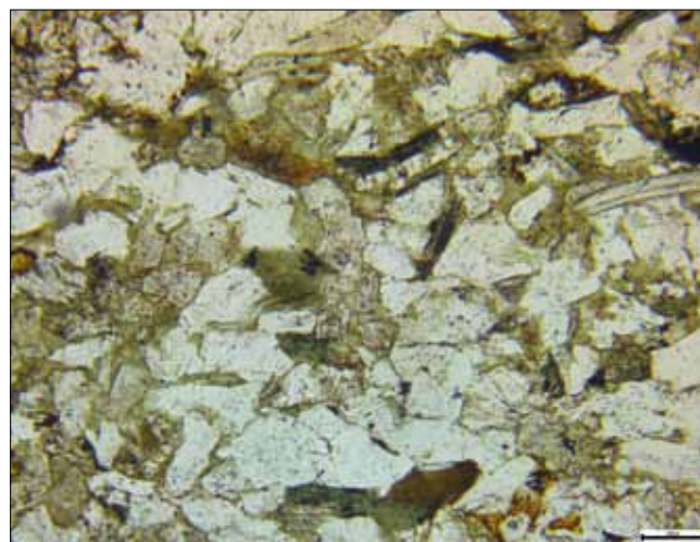
Sl. 202 Mikrofotografija litičnog arenita (N=). Uzorak: SJ 504-N 171 (skala veličine 100 mikrona), kat. br. 5
