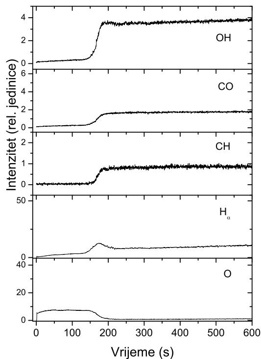
Slika 5.55: Vremensko odvijanje odabranih linija, na 120 Pa
