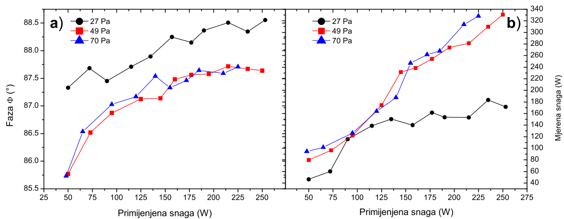
Slika 4.15: a) Faza između struje i napona b) Mjerena snazi za različite tlakove u ovisnosti o primijenjenoj snazi.
