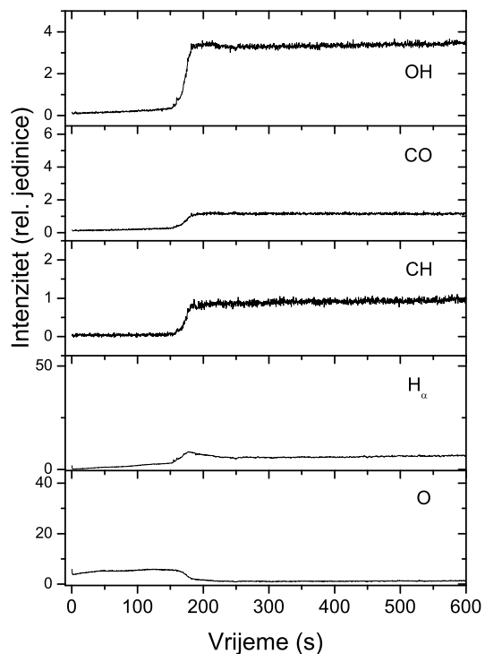
Slika 5.54: Vremensko odvijanje odabranih linija, na 100 Pa
