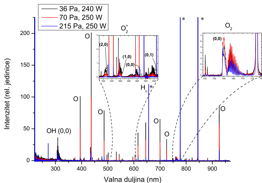
Slika 5.1: Optički emisijski spektar kisika, za tri različita tlaka, uvećani su dijelovi spektra s molekularnim vrpčama. Primijenjena snaga je 240-250 W.
