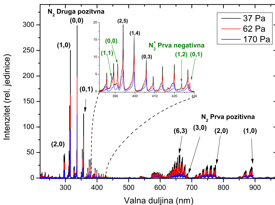
Slika 5.7: Optički emisijski spektar dušika za tri različita tlaka, a uvećan je dio spektra (382-430 nm) s molekularnom vrpcom N_2^+ (zelenom bojom i strelicama su označene ionske vrpce). Primijenjena snaga od 200 W.
