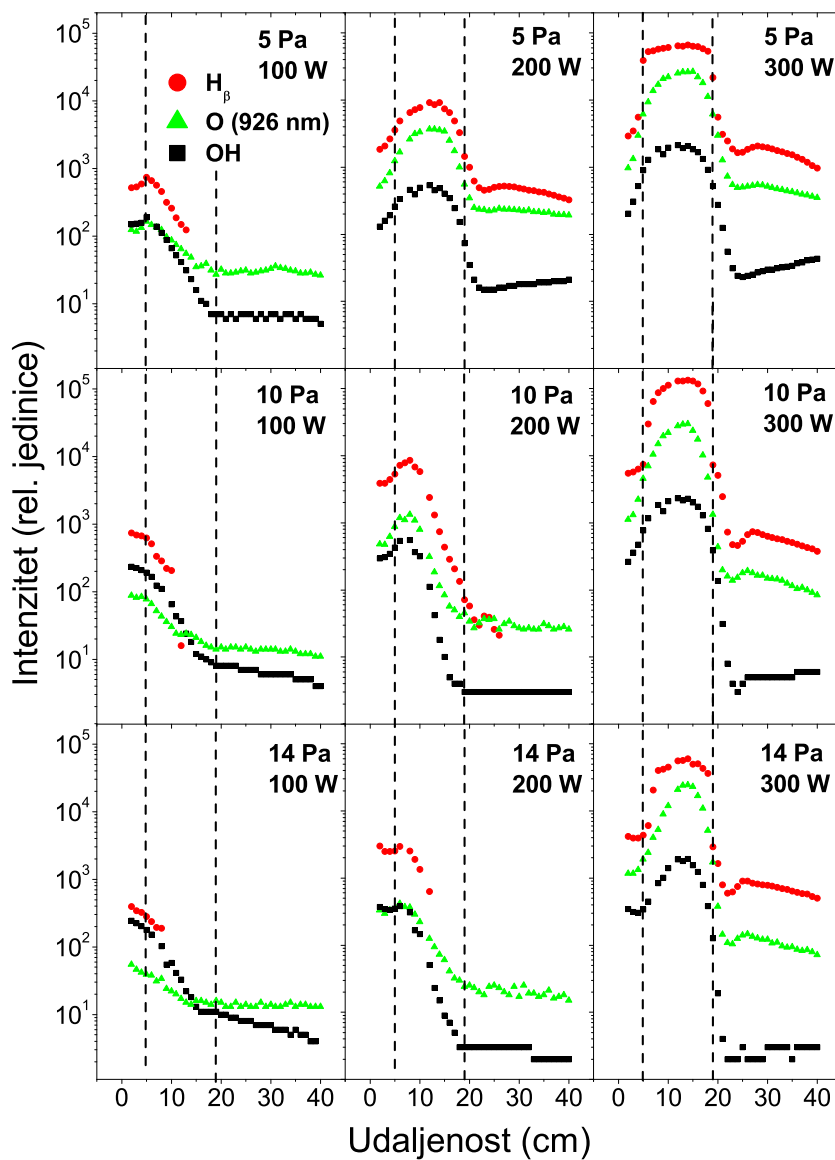
Slika 5.15: Prostorna raspodjela intenziteta za H_\beta na 486 nm, O ( 3d^5D^O - 3p^5P ) liniju na 926.3 nm i OH(0,0) na 309 nm. Tok vodene pare je slijeva nadesno, a crtkane linije označavaju poziciju zavojnice.
