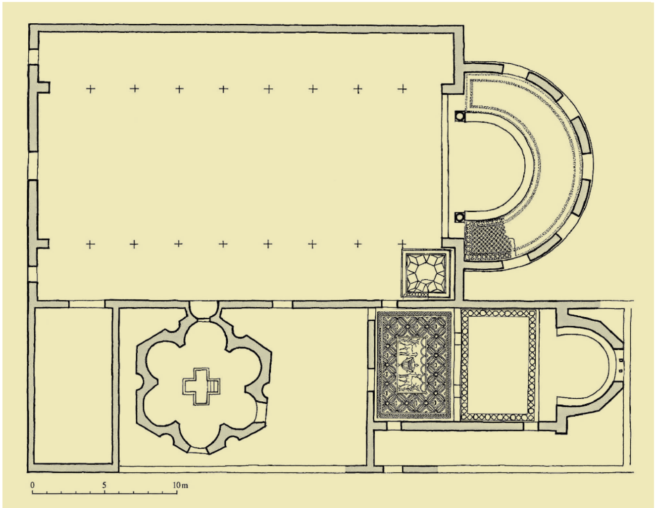
2. Tlocrt ranokršćanske katedrale u Zadru s aneksima (izvor: PAVUŠA VEŽIĆ /bilj. 28, 2005./, 37)
