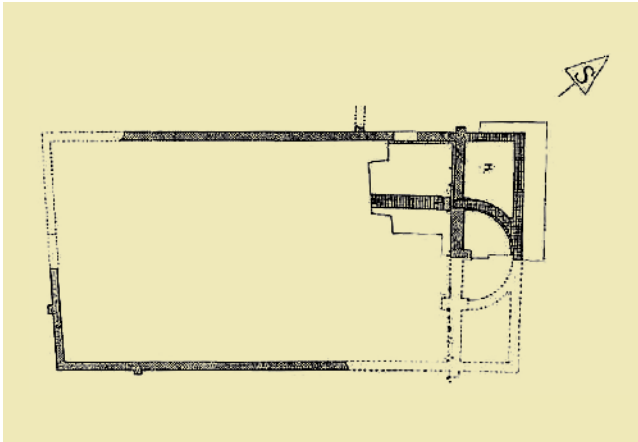
1. Tlocrt crkve u Jurandvoru na otoku Krku; slovo M. označuje poziciju mozaičnog natpisa (izvor: RANKO STARAC /bilj. 10/, 137)
