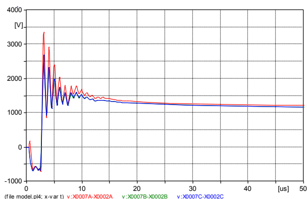
Slika 11. Napon na transformatoru, priključeni odvodnici prenapona u objektu i TR (val 100 kA, 10/350 \mu s), U_{\max}=3,343 kV
