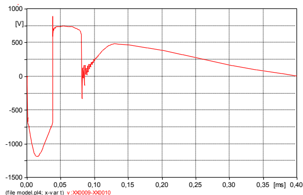
Slika 10. Napon na potrošaču, priključeni odvodnici prenapona u objektu (100 kA, 8/20 \mu s), U_{\max}=-1,187 kV
