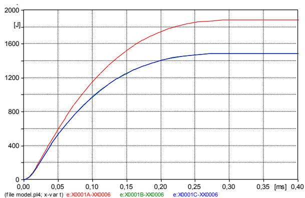
Slika 15. Energija koju apsorbiraju odvodnici prenapona u objektu (100 kA, 10/350 \mu s), E_{od1}=1,88 kJ, E_{od2}=1,49 kJ, E_{od3}=1,49 kJ
