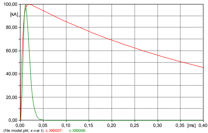
Slika 4. Strujni impuls 100 kA valnog oblika 8/20 \mu s (zeleno) i 10/350 \mu s (crveno)
