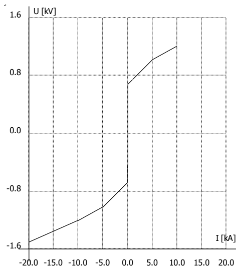
Slika 3. Strujno-naponska karakteristika NN MO odvodnika prenapona
