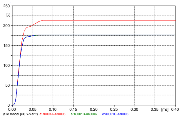
Slika 16. Energija koju apsorbiraju odvodnici prenapona u objektu (100 kA, 8/20 \mu s), E_{od1}=214,1 J, E_{od2}=176,9 J, E_{od3}=177,0 J
