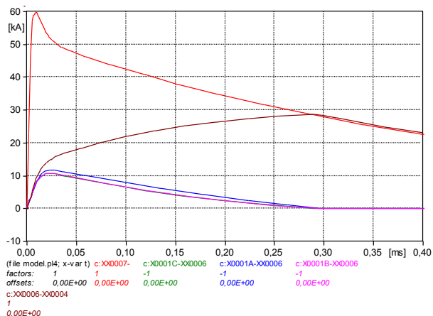
Slika 13. Struja kroz uzemljivač, odvodnike prenapona u objektu te PEN vodič (100 kA, 10/350 \mu s), I_{uzmax}=59,7 kA, I_{od1max}=11,65 kA, I_{od2max}=10,70 kA, I_{od3max}=10,70 kA, I_{PENmax}=28,59 kA
