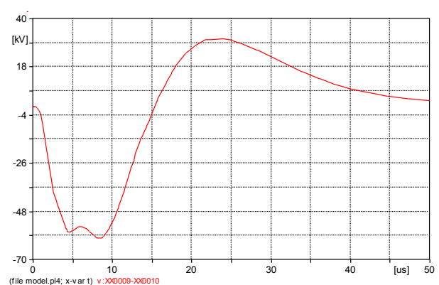
Slika 8. Napon na potrošaču, nisu priključeni odvodnici prenapona u objektu (100 kA, 8/20 \mu s), U_{max}=-60,2 kV
