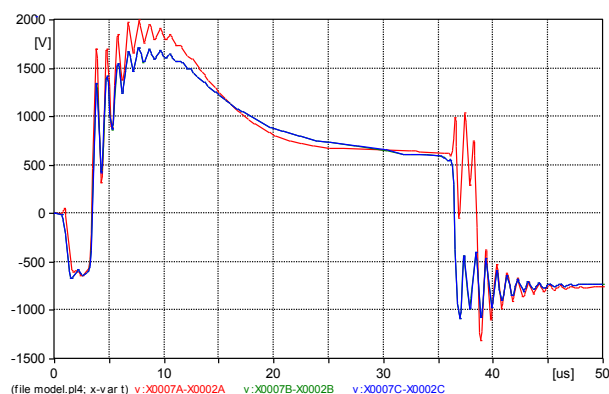
Slika 12. Napon na transformatoru, priključeni odvodnici prenapona u objektu i TR (100 kA, 8/20 \mu s), U_{\max}=1,996 kV
