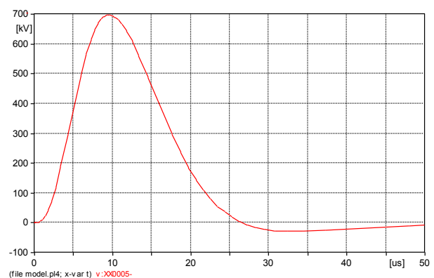
Slika 6. Napon na uzemljivaču objekta, nisu priključeni odvodnici prenapona u objektu (100 kA, 8/20 \mu s), U_{max}=697,0 kV
