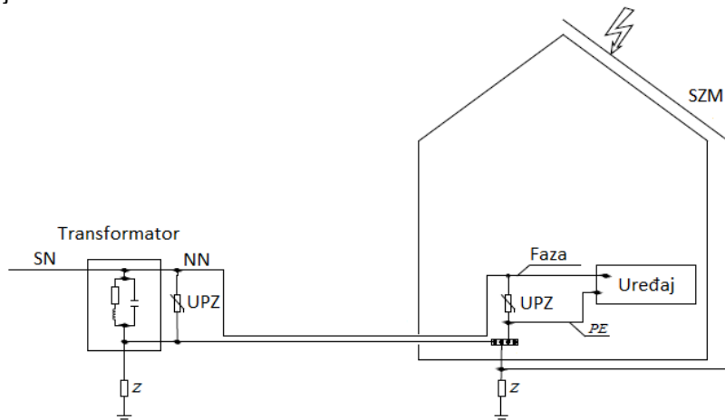
Slika 1. Pojednostavljena shema niskonaponske instalacije
