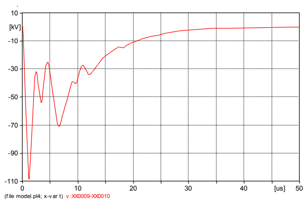
Slika 7. Napon na potrošaču, nisu priključeni odvodnici prenapona u objektu (100 kA, 10/350 \mu s), U_{max}=-108,2 kV
