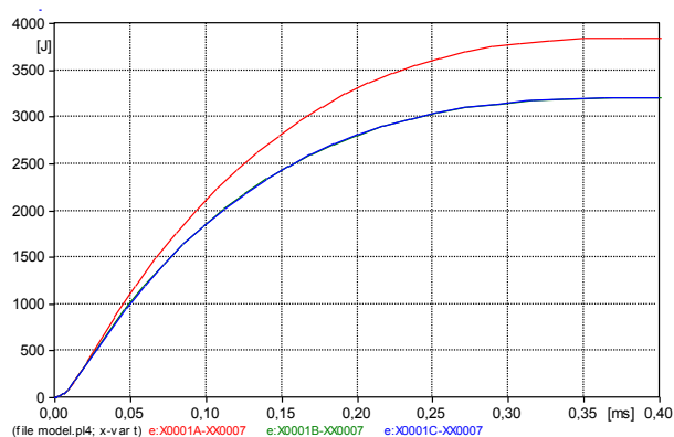
Slika 17. Energija koju apsorbiraju odvodnici prenapona u objektu (100 kA, 10/350 \mu s), E_{od1}=3,84 kJ, E_{od2}=3,20 kJ, E_{od3}=3,20 kJ
