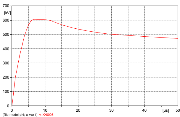
Slika 5. Napon na uzemljivaču objekta, nisu priključeni odvodnici prenapona u objektu (100 kA, 10/350 \mu s), U_{max}=607,6 kV
