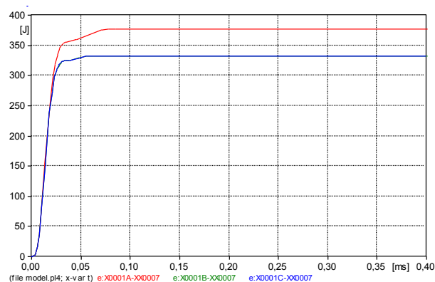
Slika 18. Energija koju apsorbiraju odvodnici prenapona u objektu (100 kA, 8/20 \mu s), E_{od1}=377,0 J, E_{od2}=332,4 J, E_{od3}=332,6 J
