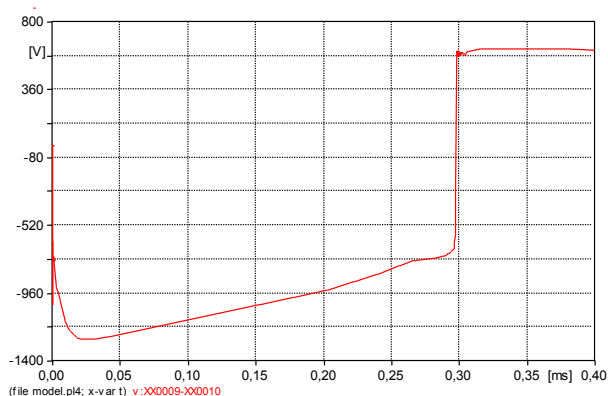
Slika 9. Napon na potrošaču, priključeni odvodnici prenapona u objektu (100 kA, 10/350 \mu s), U_{\max}=-1,260 kV
