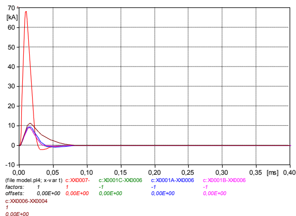
Slika 14. Struja kroz uzemljivač, odvodnike prenapona u objektu te PEN vodič (100 kA, 8/20 \mu s), I_{uzmax}=68,3 kA, I_{od1max}=9,54 kA, I_{od2max}=9,00 kA, I_{od3max}=9,01 kA, I_{PENmax}=11,27 kA
