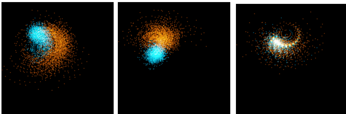
iteracija 21 dobrota: 6.29
