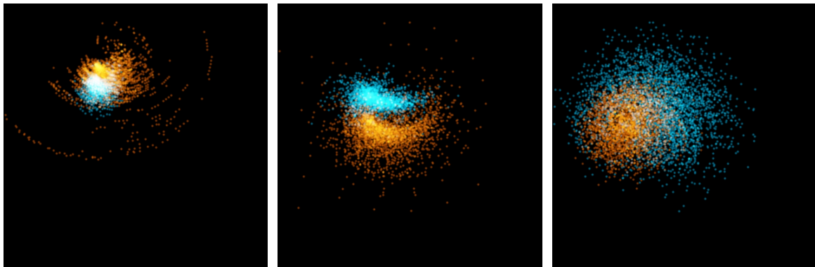
iteracija 13 dobrota: 11.63
