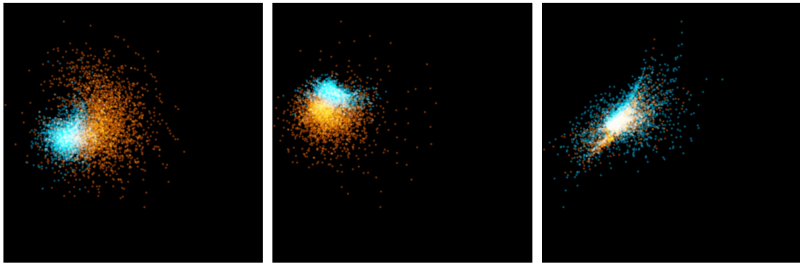
iteracija 5 dobrota: 3.48
