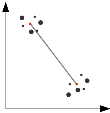
Slika 4.10 Euklidska udaljenost
