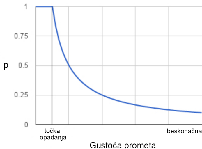
Slika 3.4. Vjerojatnost razaslanja poruke u ovisnosti o gustoći prometa
