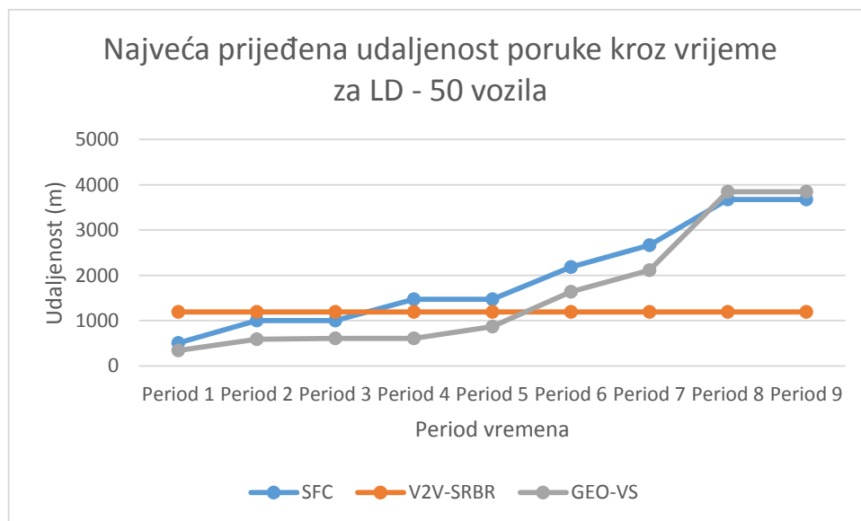
Slika 3.51. Usporedba najveće prijeđene udaljenosti poruka za LD gustoću prometa GEO-VS algoritma sa SCF i V2V-SRBR modelima komunikacije
