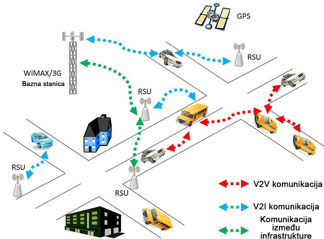
Slika 2.3. Prikaz komunikacije u ad-hoc mrežama vozila 1
