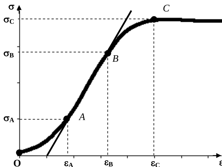
Slika 5.12. Graf ovisnosti deformacije o naprezanju pri tlačnom djelovanju sile paralelno s vlakancima u longitudinalnom smjeru: \sigma_A – minimalno elastično naprezanje, \epsilon_A – minimalna elastična deformacija, \sigma_B – maksimalno elastično naprezanje, \epsilon_B – maksimalna elastična deformacija, \sigma_C – maksimalno naprezanje, \epsilon_C – deformacija pri maksimalnom naprezanju
