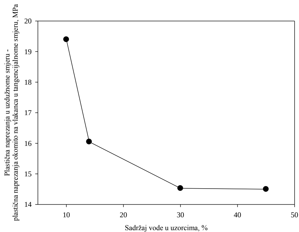
Slika 8.7. Dijagram ovisnosti razlike plastičnih naprezanja u uzdužnom smjeru i okomito na vlakanca u tangencijalnom smjeru o sadržaju vode u uzorcima
