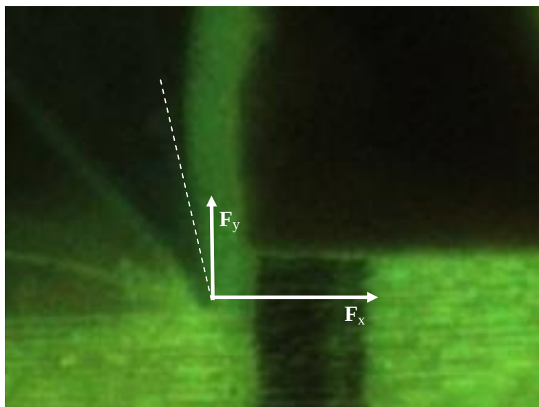
Slika 7.8. Prikaz izmjerenih komponenti sile: \mathbf{F}_x – sila rezanja, \mathbf{F}_y – odzivna sila
