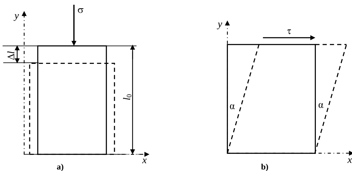
Slika 5.9. Shematski prikaz nastanka linijskih i kutnih deformacija: a) linijska deformacija ( \sigma – tlačno naprezanje, l_0 – početna duljina tijela, \Delta l – promjena duljine zbog tlačnih naprezanja) i b) kutna deformacija ( \tau – smično naprezanje, \alpha – kut za koji se tijelo deformira zbog djelovanja smičnih naprezanja)
