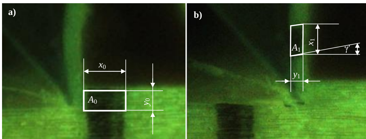
Slika 6.2. Proces plastične deformacije strugotine pri ortogonalnom rezanju drva: x_0 – duljina neodrezane strugotine, y_0 – debljina neodrezane strugotine, x_1 – duljina odrezane strugotine, y_1 – debljina odrezane strugotine, A_0 – površina neodrezane strugotine, A_1 – površina odrezane strugotine, \gamma – kut smicanja
