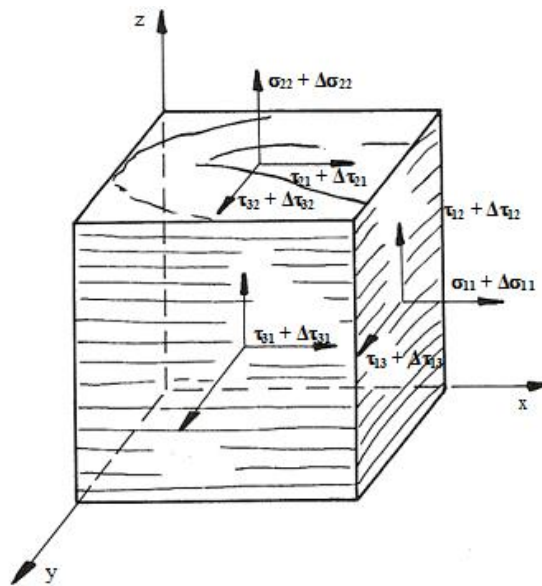
Slika 5.8. Shematski prikaz komponenata tenzora naprezanja
