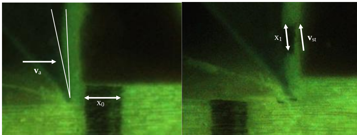
Slika 6.5. Definiranje kinematičkih veličina ortogonalnog rezanja: x_0 – duljina dijela neodrezane strugotine, x_1 – duljina dijela odrezane strugotine, v_a – brzina alata, v_{st} – brzina strugotine
