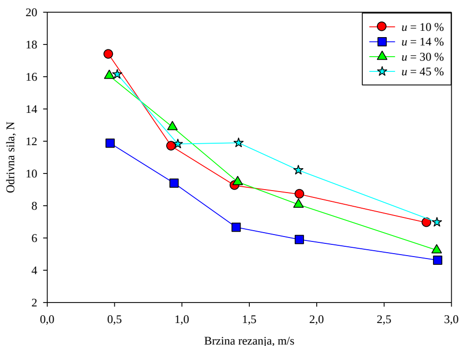
Slika 8.8. Dijagram ovisnosti srednje vrijednosti odzivne sile o brzini rezanja za sadržaje vode u uzorcima u = (10, 14, 30 \text{ i } 45) \%
