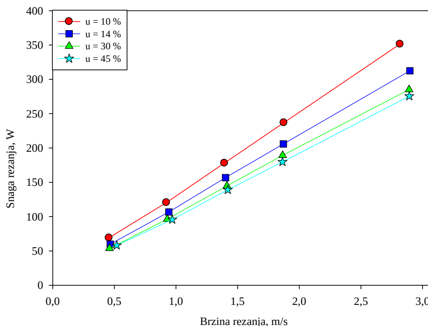
Slika 8.10. Dijagram ovisnosti srednje vrijednosti snage rezanja o brzini rezanja za sadržaje vode u uzorcima u = (10, 14, 30 \text{ i } 45) \%
