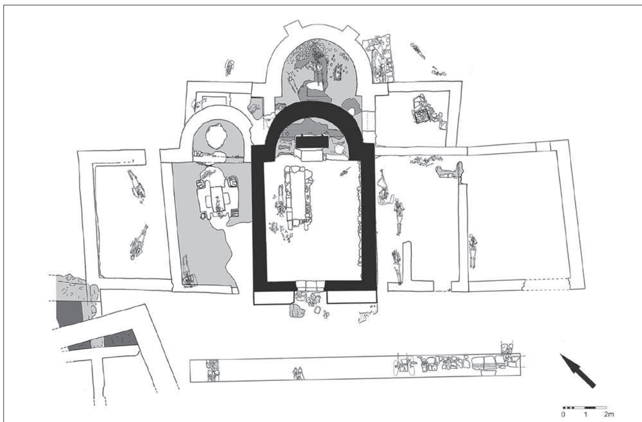
Sl. 3. Sakralni kompleks Sv. Marije na Tarcu – tlocrt istraženih ostataka arhitekture s kasnijim grobovima (prema M. Zornija izradio M. Košta, Pixel g.t.o., Zadar)
