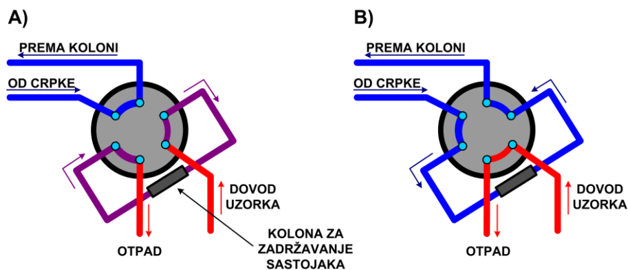
Slika 18. Osnovne faze online pretkoncentriranja analita:
