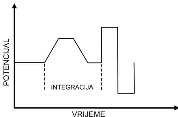
Slika 44. Puls u integriranoj amperometriji.
