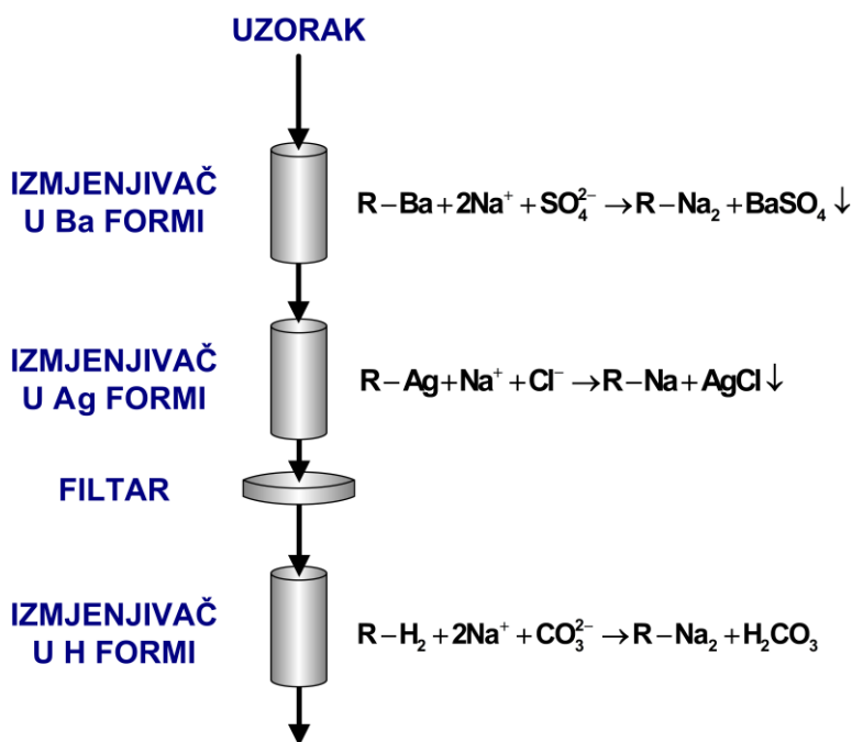
Slika 17. Uklanjanje različitih sastojaka iz matrice serijskim povezivanjem niza kolona.
