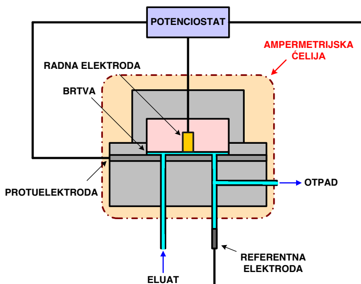
Slika 41. Ampermetrijski detektor.
