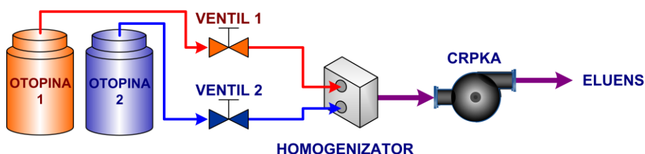
Slika 8. Sustav miješanja eluensa pri niskom tlaku.
