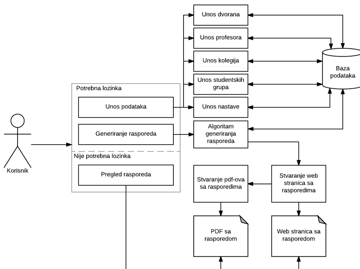
Slika 11. Hodogram korištenja
