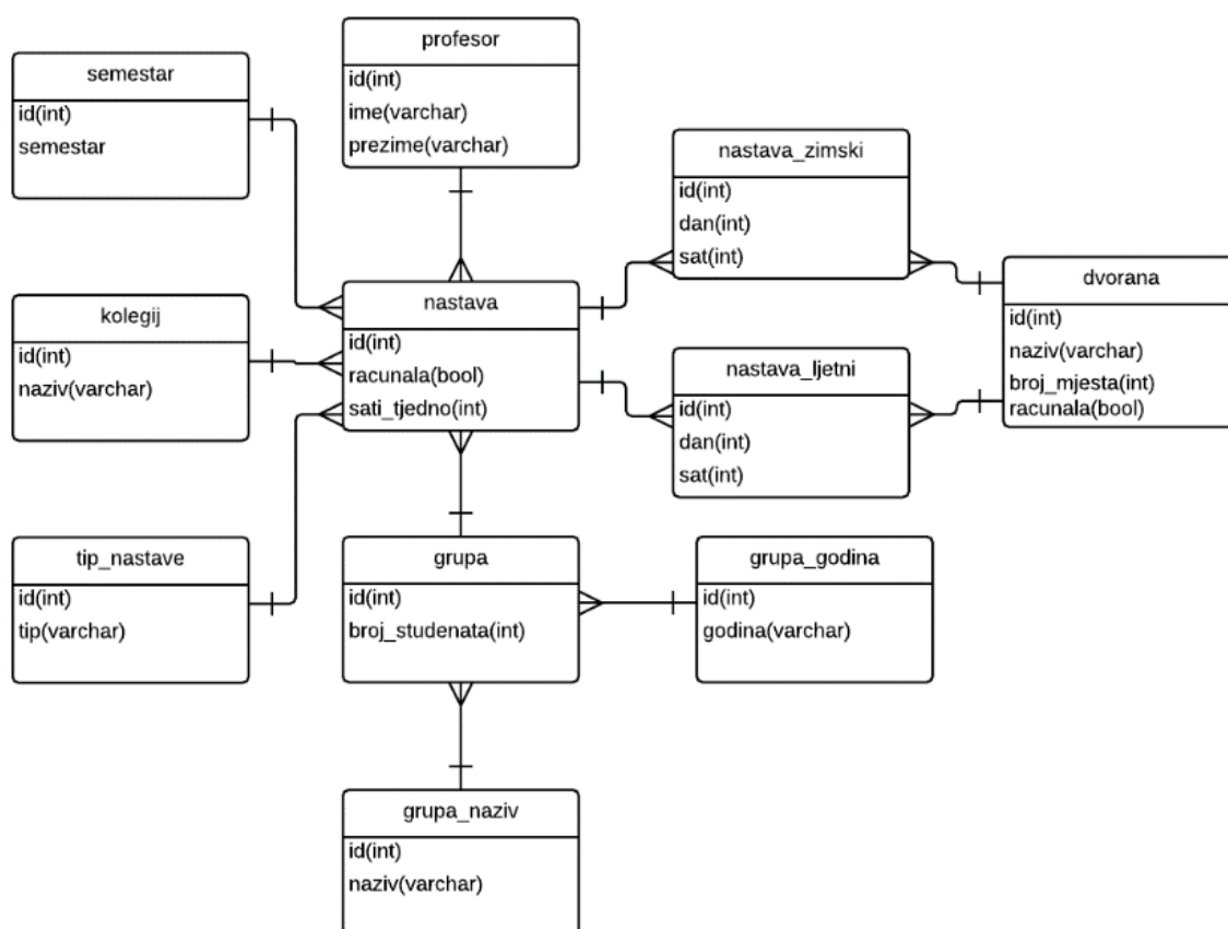
Slika 21. Baza podataka
