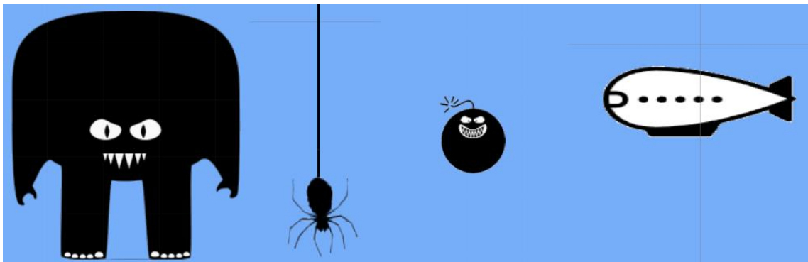
Slika 15.Objekti neprijatelji.
