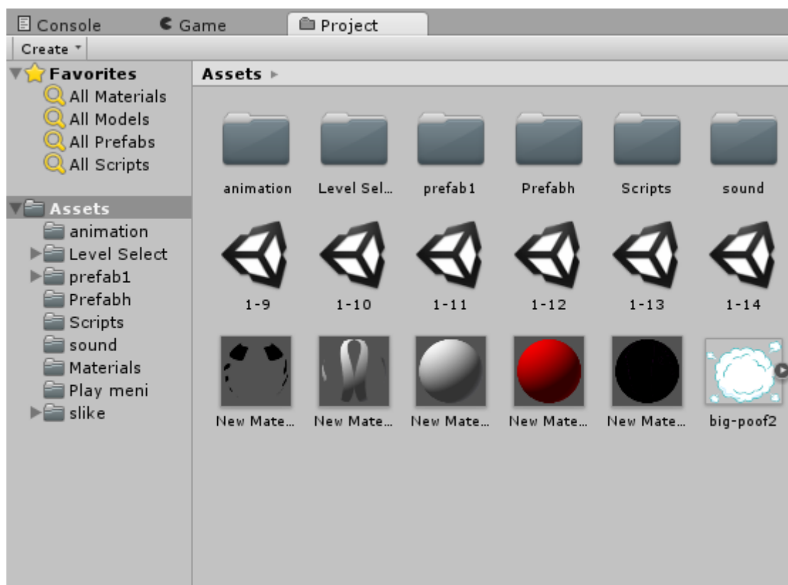
Slika 6: Preglednik projekta
