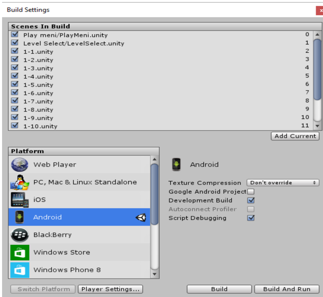
Slika 7: Izbornik formata
