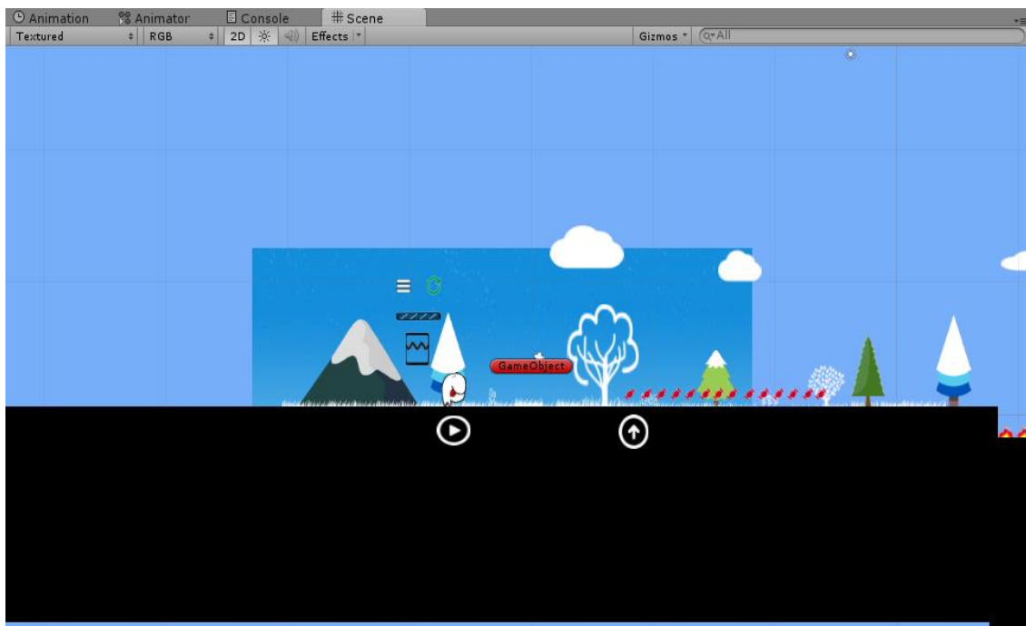
Slika 4 Preglednik scene
