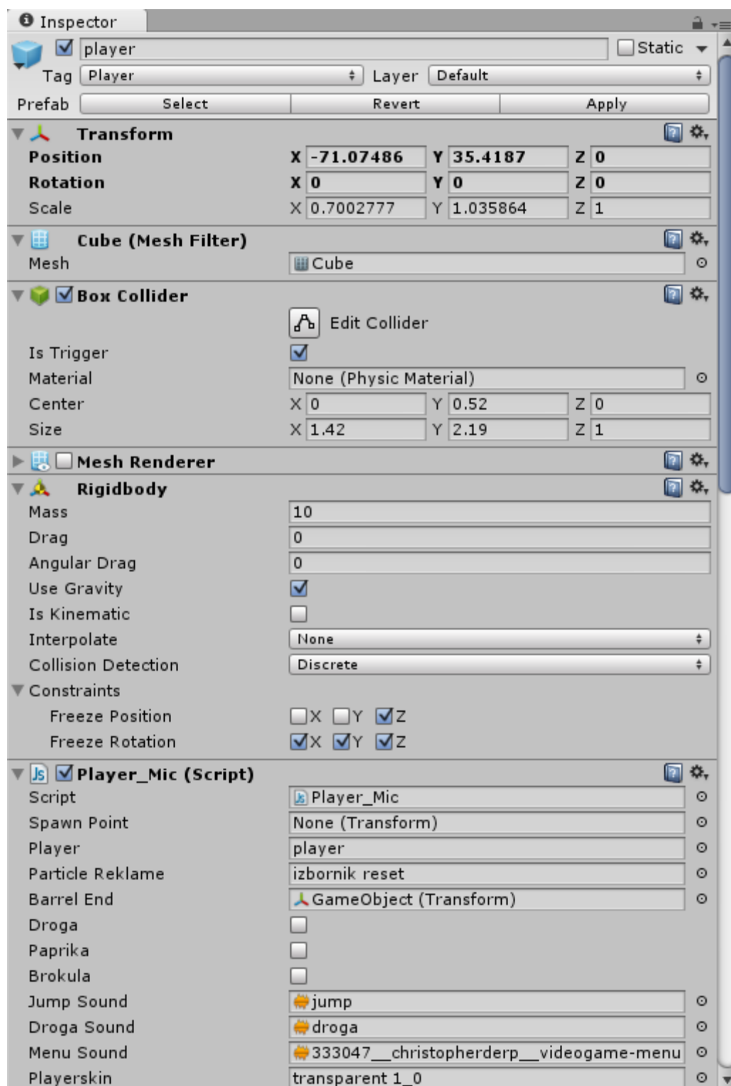
Slika 5: Inspektor
