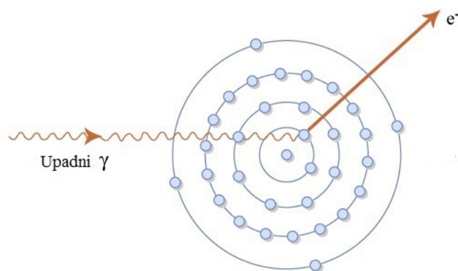
Slika 2.10: Fotoelektrični učinak.
