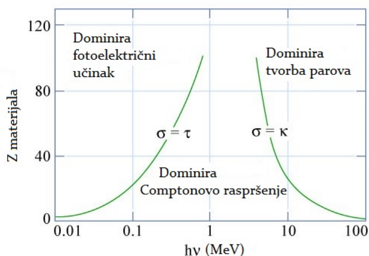
Slika 2.9: Vjerojatnost procesa ovisno o energiji upadnog fotona i atomskom broju materijala. Zelene linije pokazuju za koje su vrijednosti atomskog broja apsorbera Z i energije fotona h\nu susjedni procesi jednako vjerojatni.
