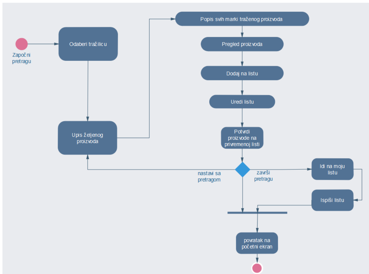
Slika 10. Prikaz aktivnosti pretrage (izvor: autor, Edraw Max)
