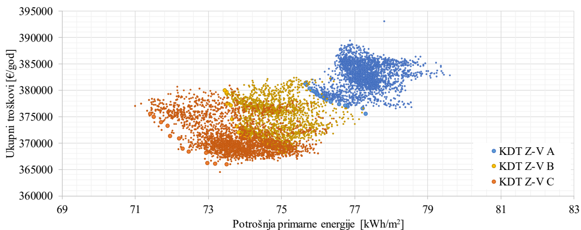
Slika P7.6 Rezultati optimizacije tehničkih sustava kompresijskih dizalica topline zrak-voda (južni Jadran)
