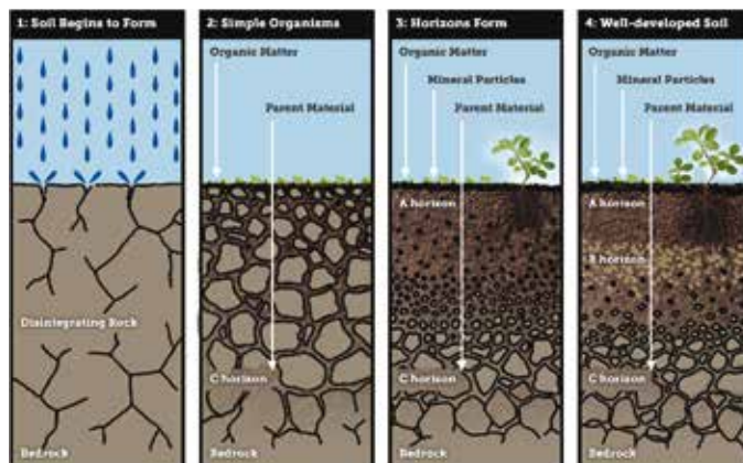
Slika 9: Trošenje stijena, stvaranje i strukturiranje tla ( https://learn.weatherstem.com/modules/learn/lessons/85/06.html )
