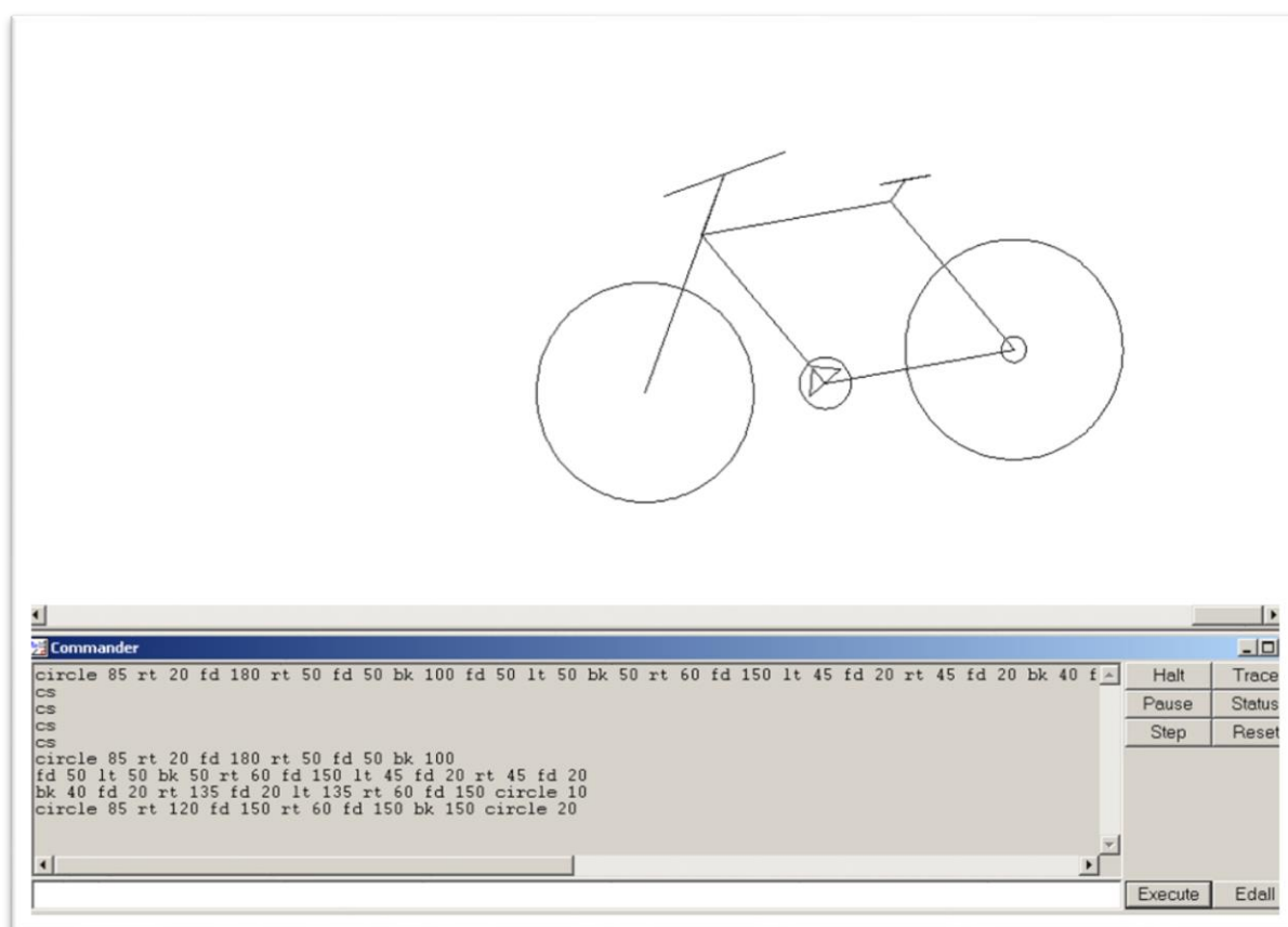
Slika 17. MSWLogo
