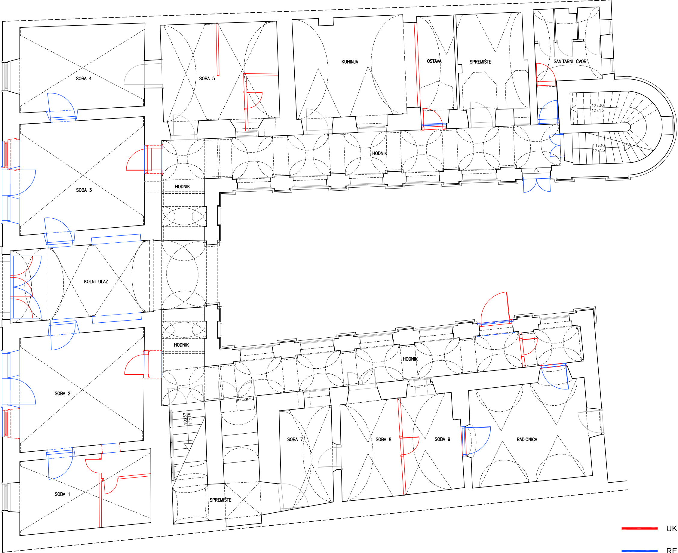
List 6 - Prijedlog konzervatorskih smjernica _ prizemlje
