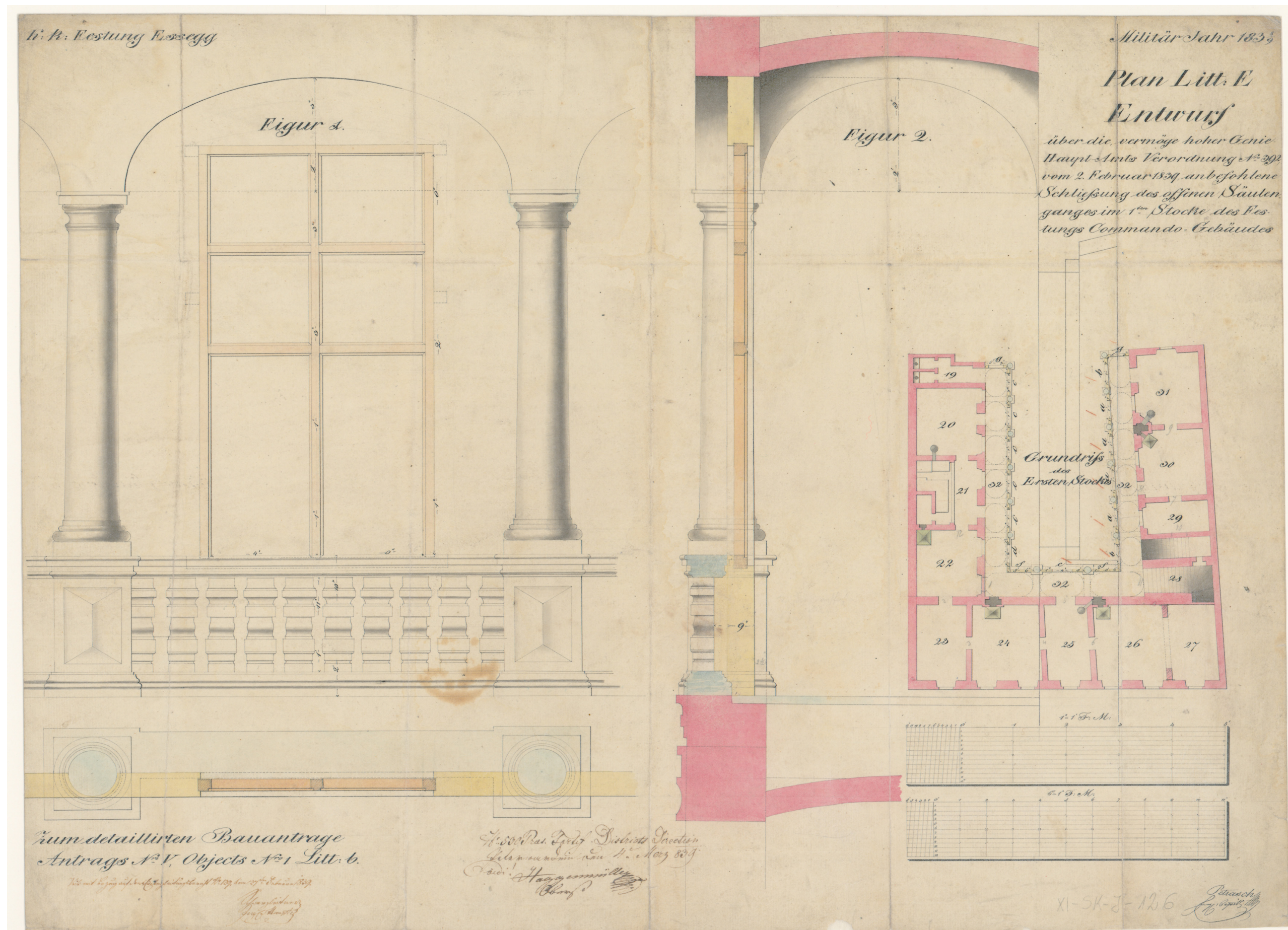
Nacrt zatvaranja dvorišnih trijemova na katu, 1838. (Izvor: NSK, Zbirka Franječić, XI-SK-J-126)
