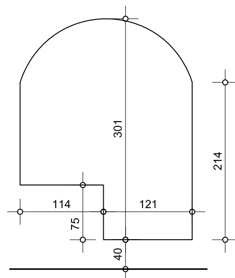
DUĆANSKI OTVOR - GRADJEVINSKE MJERE
