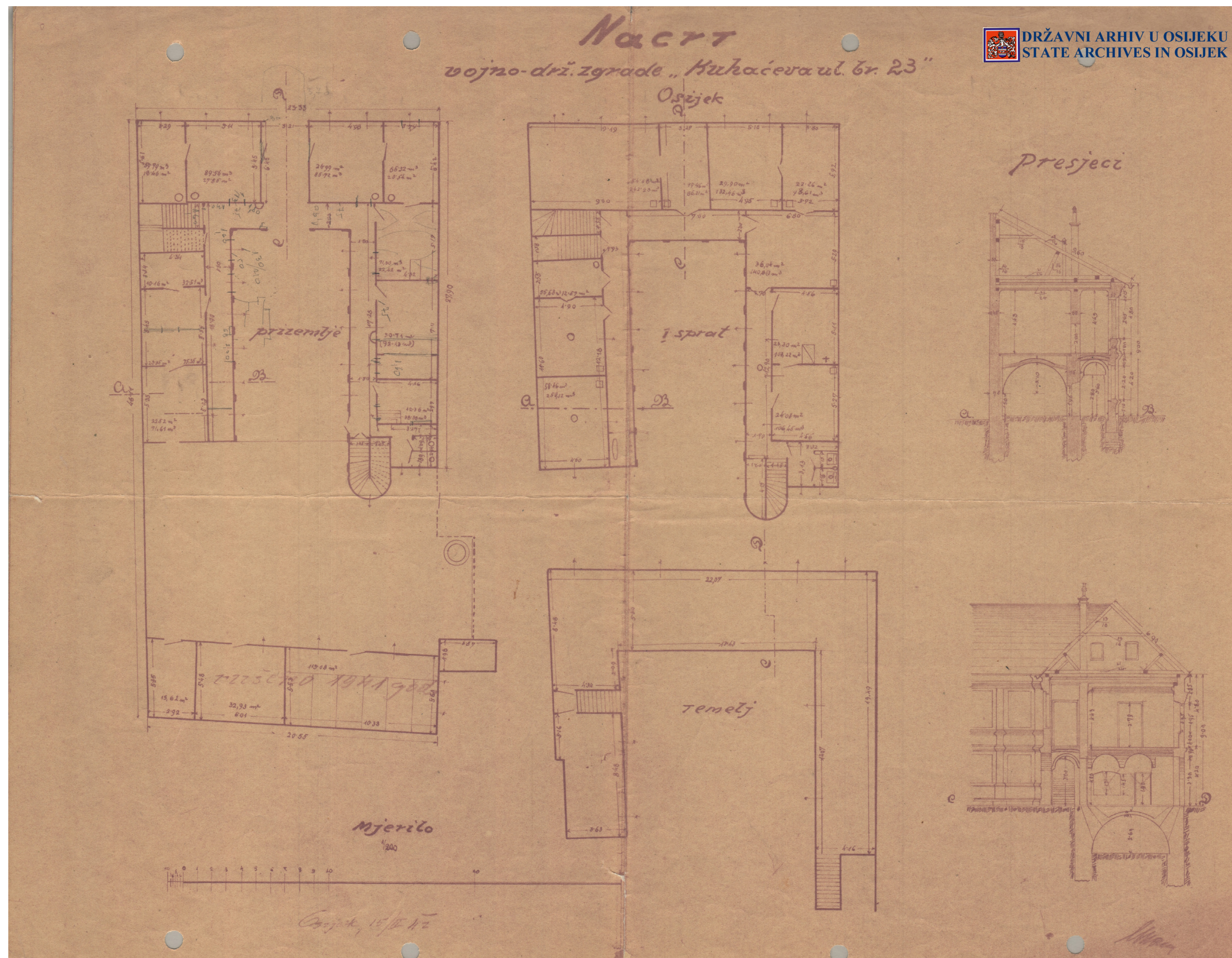
Nacrt kuće, 1942. (Izvor: HR-DAOS-6.31.1 75_23_5)
