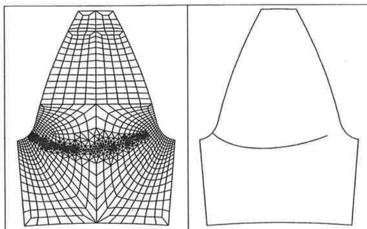
Sl. 6. Pot širjenja razpoke v zobnem korenu zobnika Fig. 6. Crack propagation path in a gear tooth root
