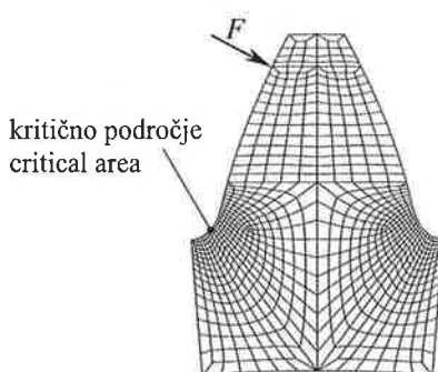
Sl. 3. Model končnih elementov Fig. 3. Finite element model
