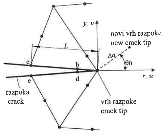
Sl. 2. Trikotni četrtinski elementi okrog vrha razpoke Fig. 2. Triangular quarter-point elements around crack tip
