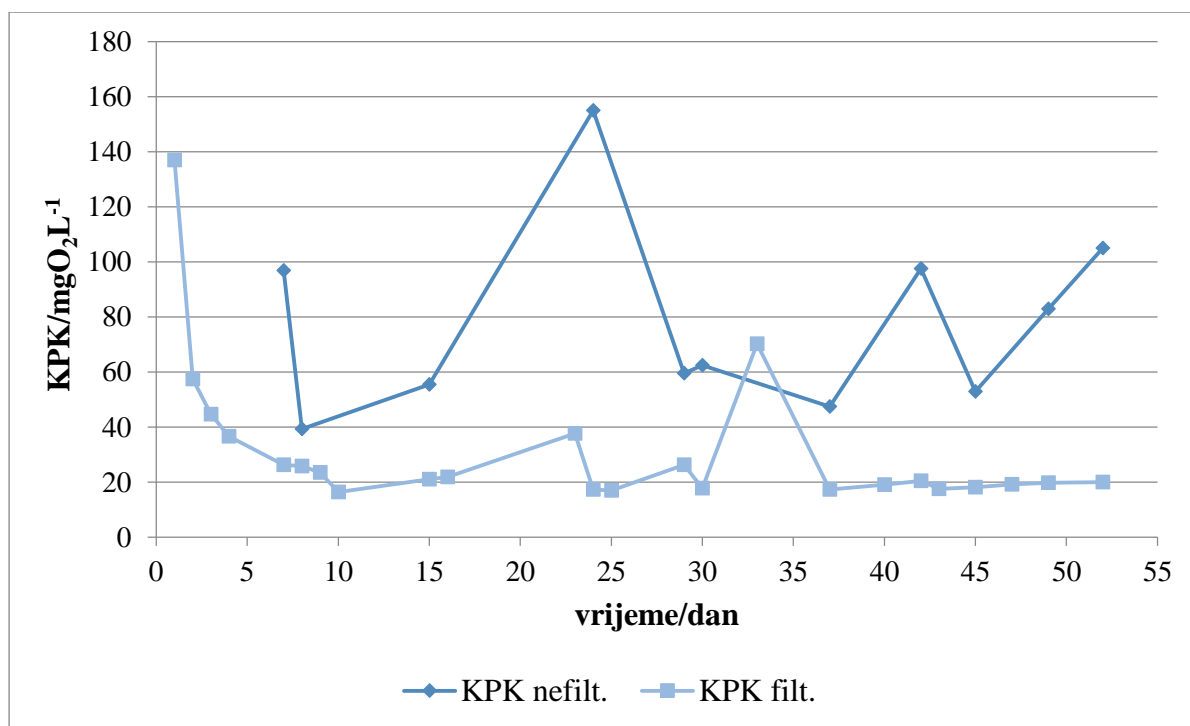
Slika 20. KPK efluenta Pokusa 2
