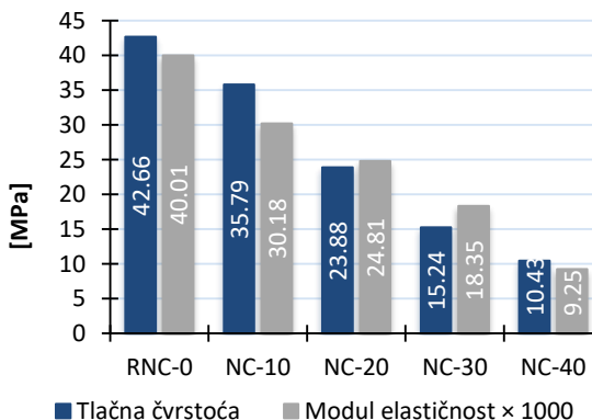
Slika 1. a) Postavke ispitivanja odnosa naprezanja i deformacije; b) Rezultati ispitivanja tlačne čvrstoće i modula elastičnosti na betonskim kockama.
