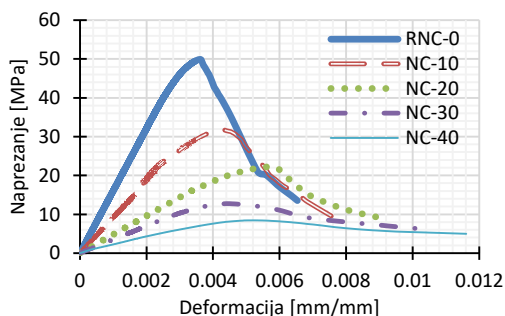
Slika 2. a) \sigma - \varepsilon krivulje za normalan beton bez gume (RNC-0-500) i normalan beton sa 10%, 20%, 30% i 40% GG; b) Ispitani betonski valjci
