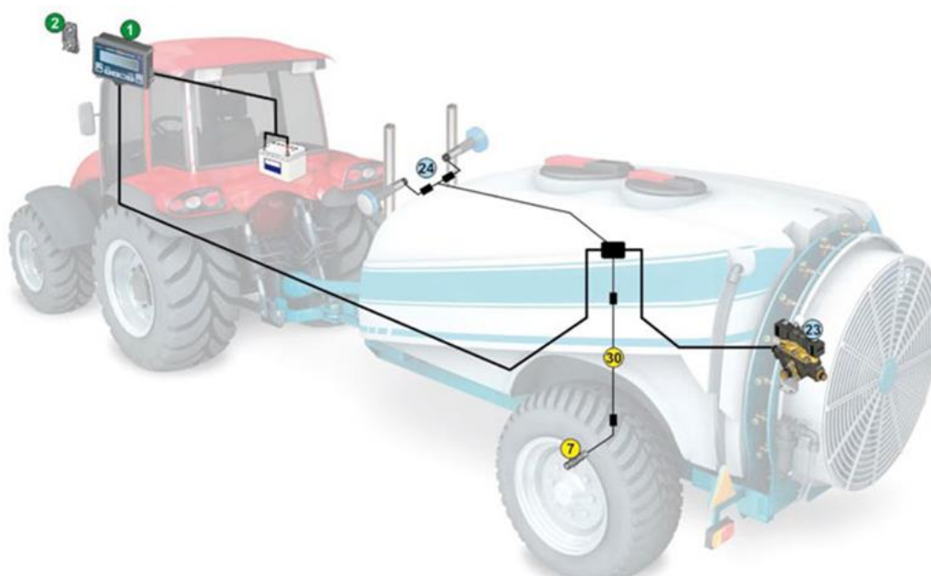
Slika 6. Shema senzorskog sustava na raspršivaču (Izvor: https://www.spritzenteile.de )
