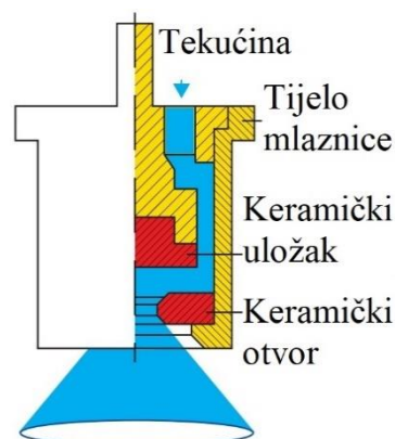
Slika 11. Mlaznica Lechler TR8002C
