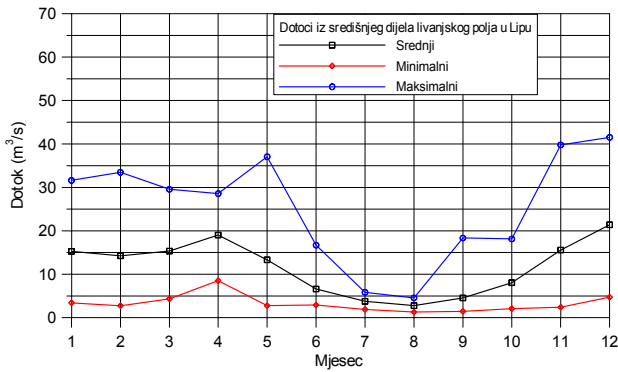
Slika 4: Srednji mjesečni dotoci u Lipu i Buško Blato u razdoblju 1975-1999. g.
