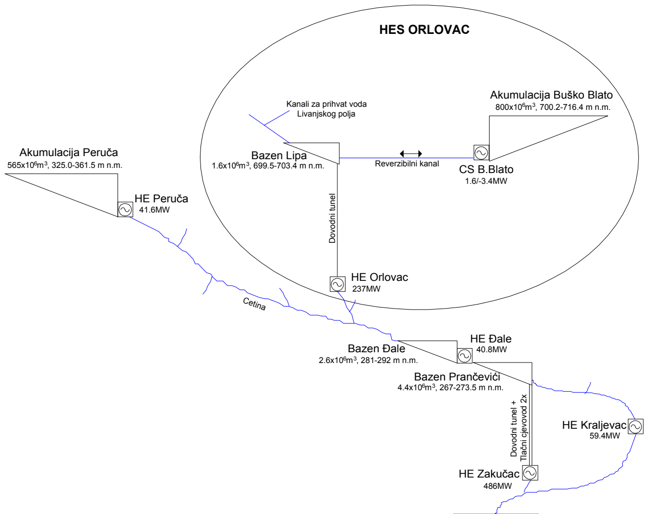
Slika 2: Položaj HES-a Orlovac u okviru HES-a Cetine
