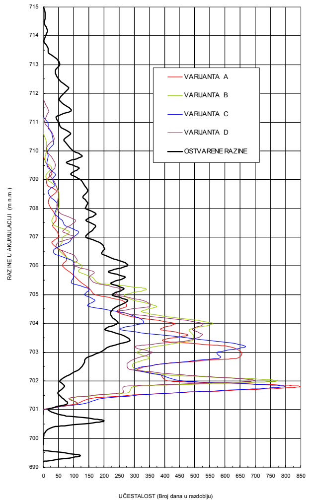
Slika 12: Učestalost razina u ak. Buško Blato
