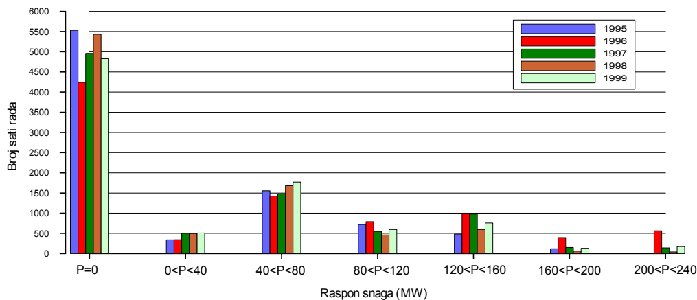
Slika 8: Raspon angažiranih snaga HE Orlovac u periodu 1995-1999.
