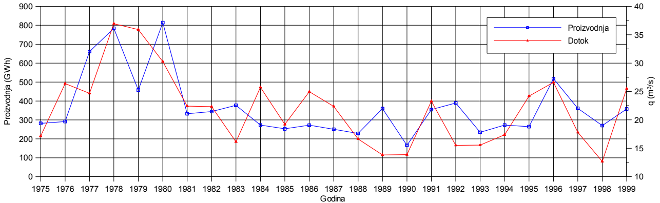
Slika 5: Proizvodnja HE Orlovac i prosječni dotoci (Lipa+Buško Blato) u razdoblju 1975-1999. g.
