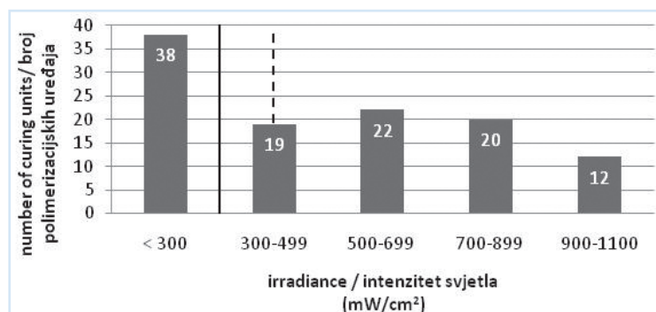
Slika 1. Distribucija polimerizacijskih uređaja prema izmjerenom intenzitetu svjetla – vertikalne crte predstavljaju minimalne operative intenzitete prema različitim autorima: puna crta – 300 mW/cm 2 , ISO standard (22); isprekidana crta – 400 mW/cm 2 , prema autorima Yapu i Seneviratnu (21).
